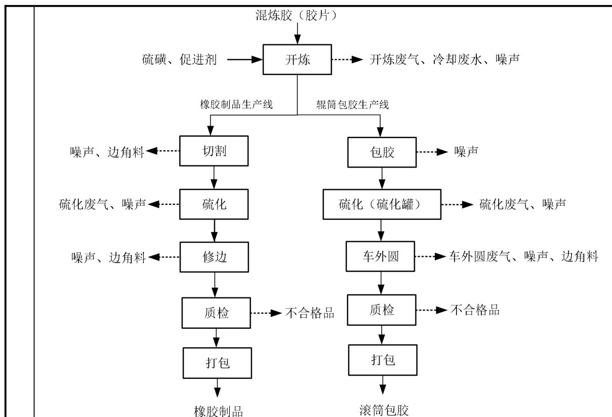
图 2-2 橡胶制品块、辊筒包胶工艺流程及产污环节图
