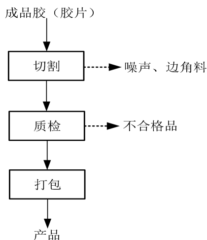
图 2-3 夹布橡胶板工艺流程及产污环节图
