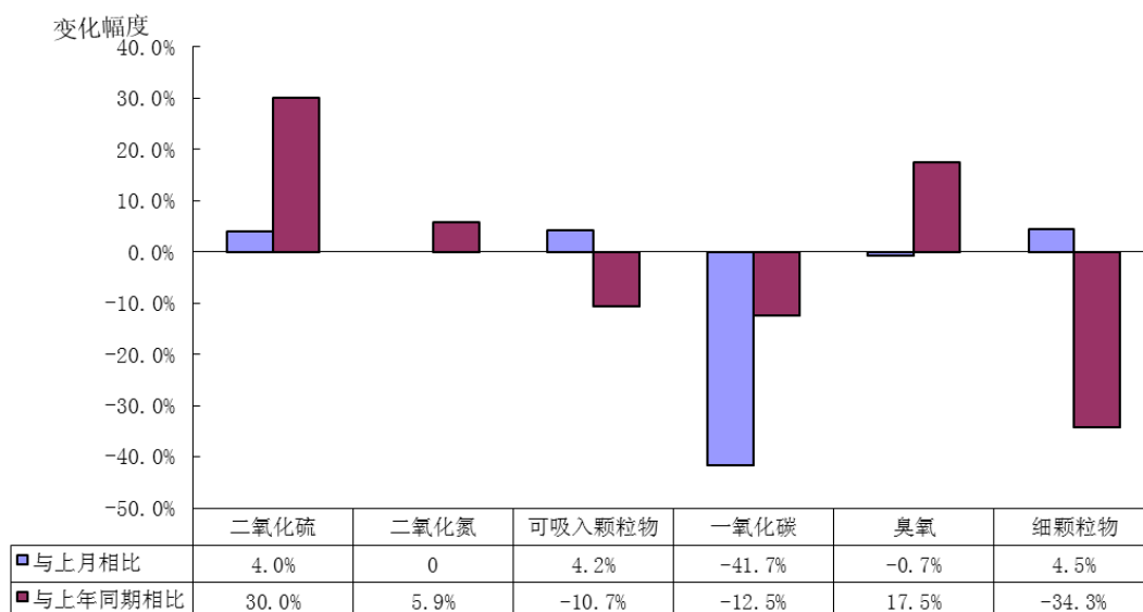
图4-1 2016年7月份各项污染物中心城区浓度均值与历史同比的变化幅度
