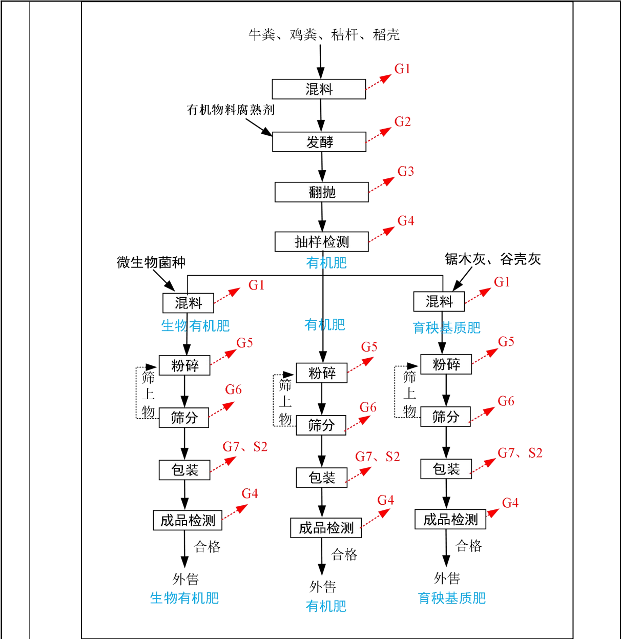
图 2-3 工艺流程及产污节点图
