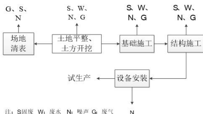
图 3.2-1 施工期工艺流程及污染节点图
