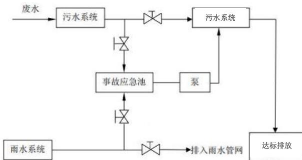
图 7.6-1 事故状态下厂区排水与外部水体的切断措施示意图
