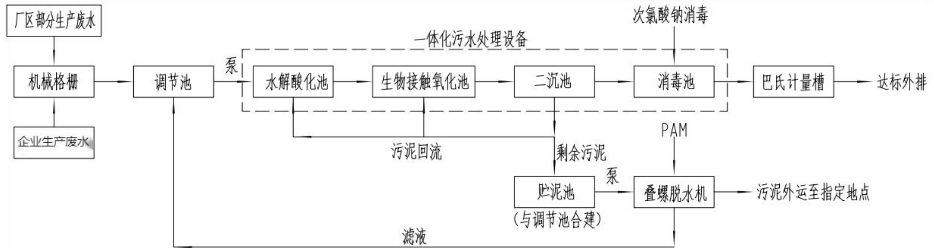
图 3.3-1 项目废水处理工艺流程图
