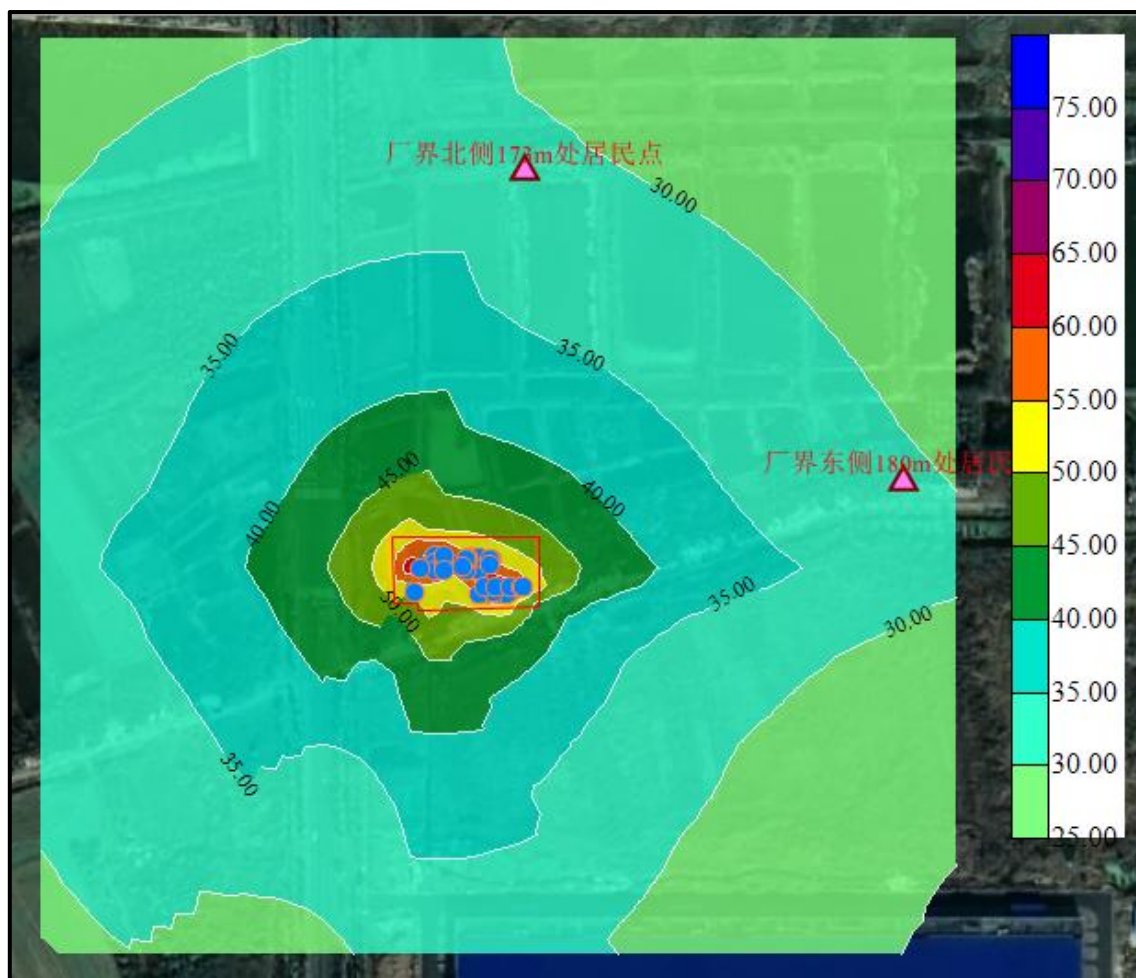
图 5.8-1 项目厂界噪声预测结果图
