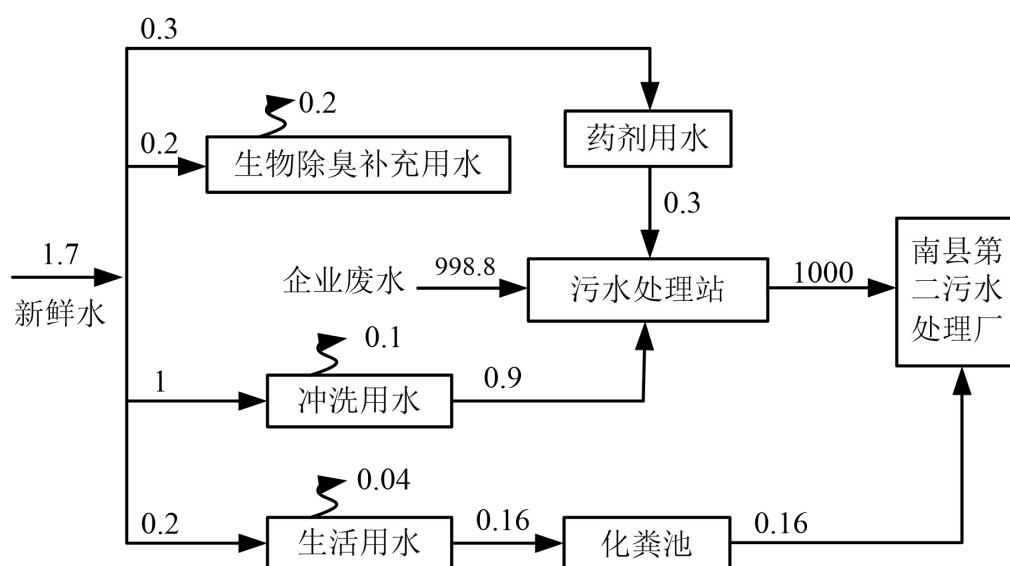
图 3.1-3 项目水平衡图 ( \text{m}^3/\text{d} )
