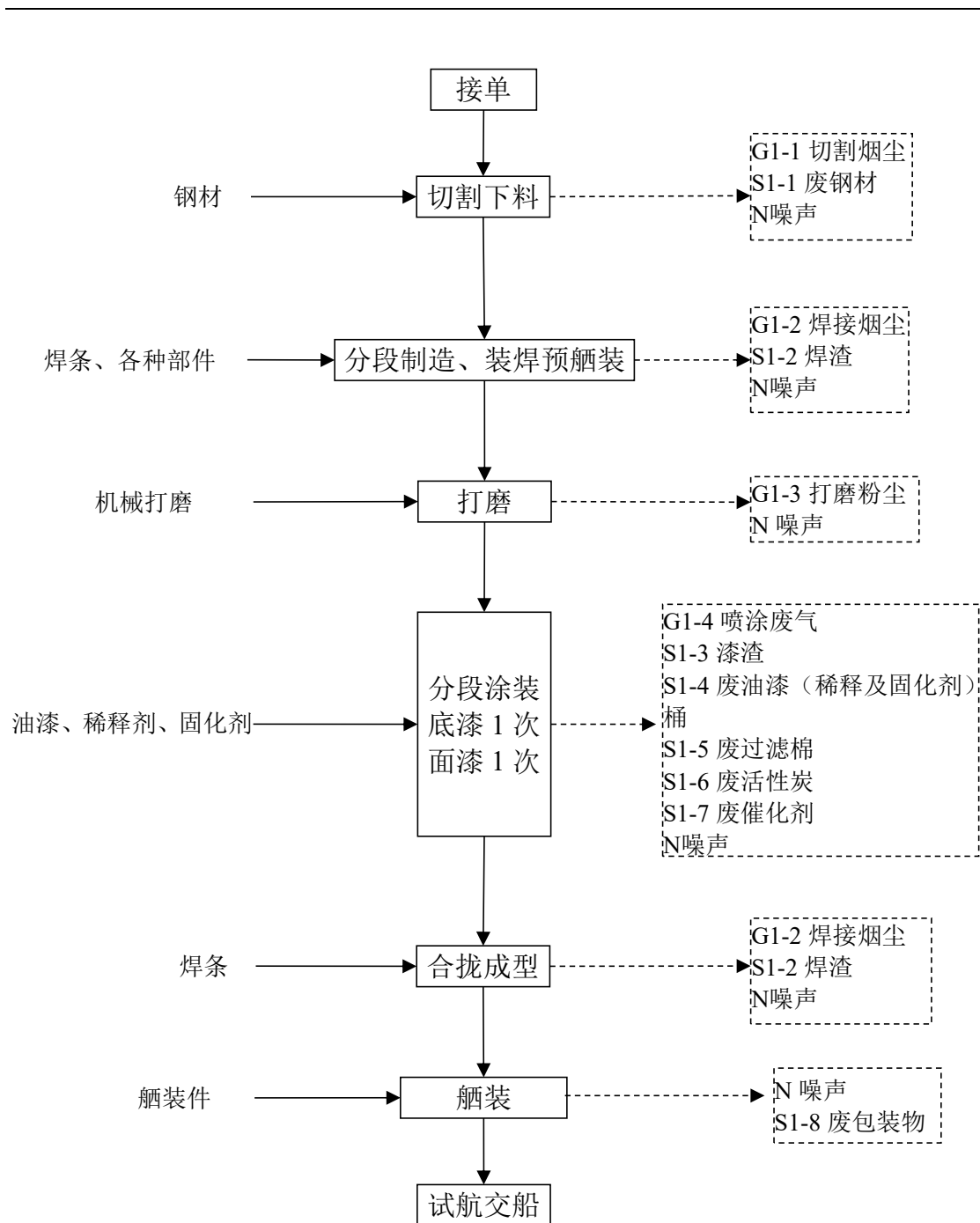
图3.4-1金属船舶生产工艺流程及产污节点图
