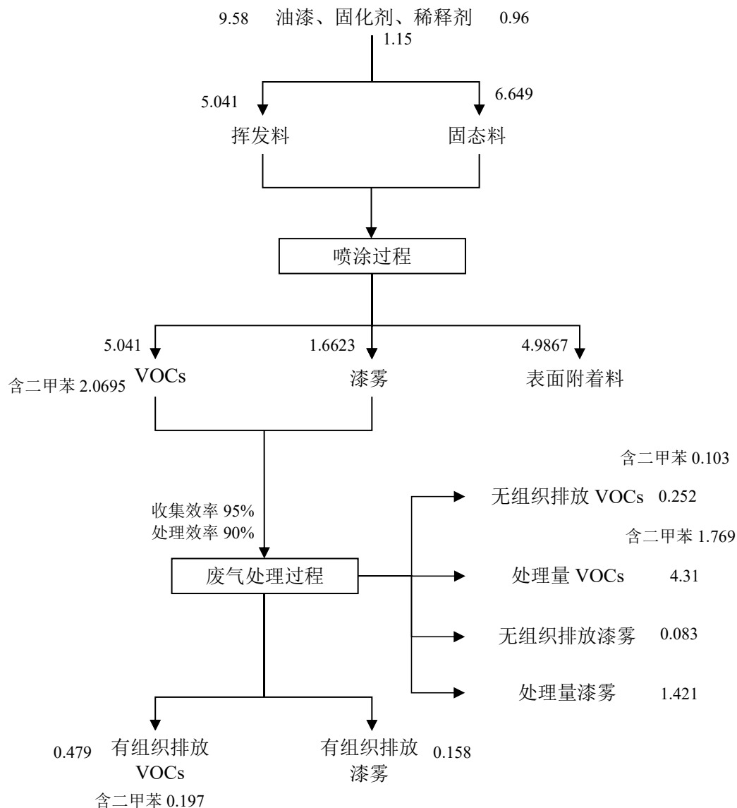
图3.4-4项目油漆及 VOCs 平衡图
