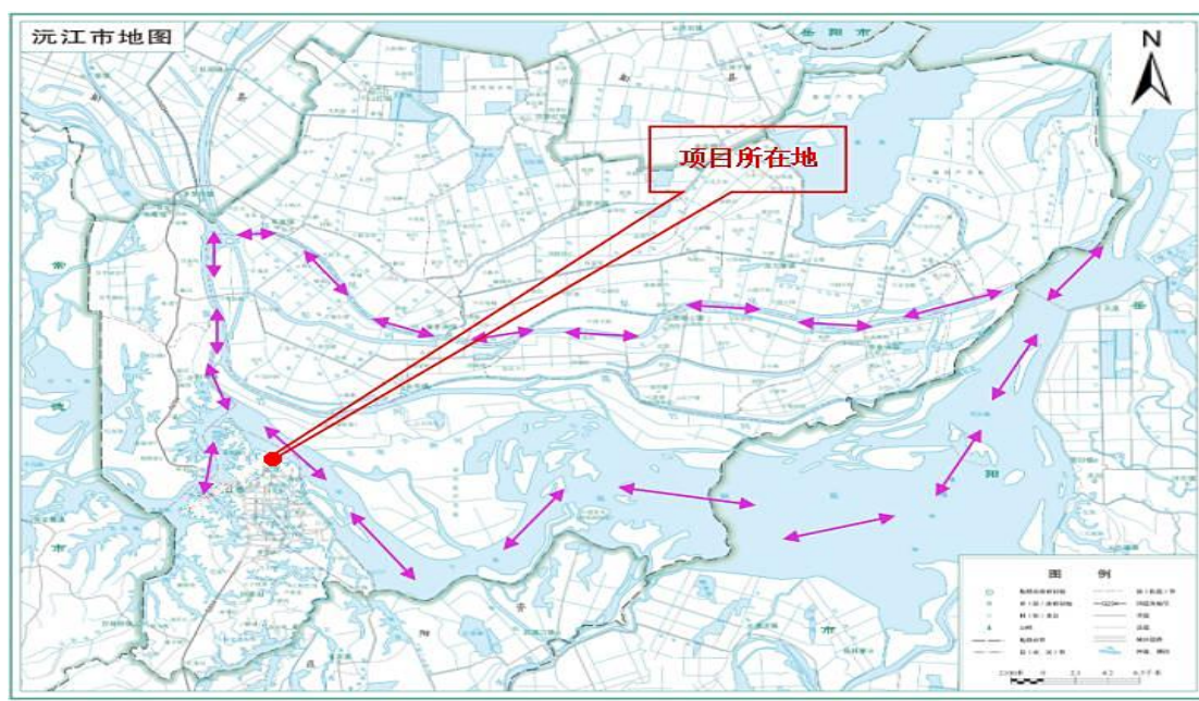
长江江豚洄游线路示意图
