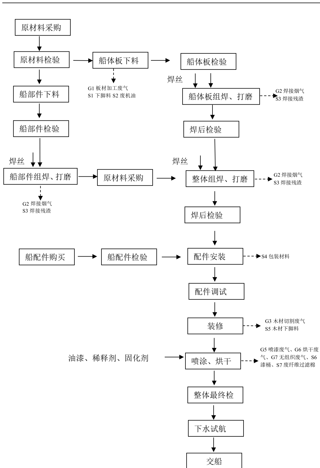
图 3.1-3 工艺流程及产污节点图
