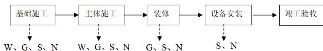
图 3.3-1 施工期工艺流程及排污节点图
