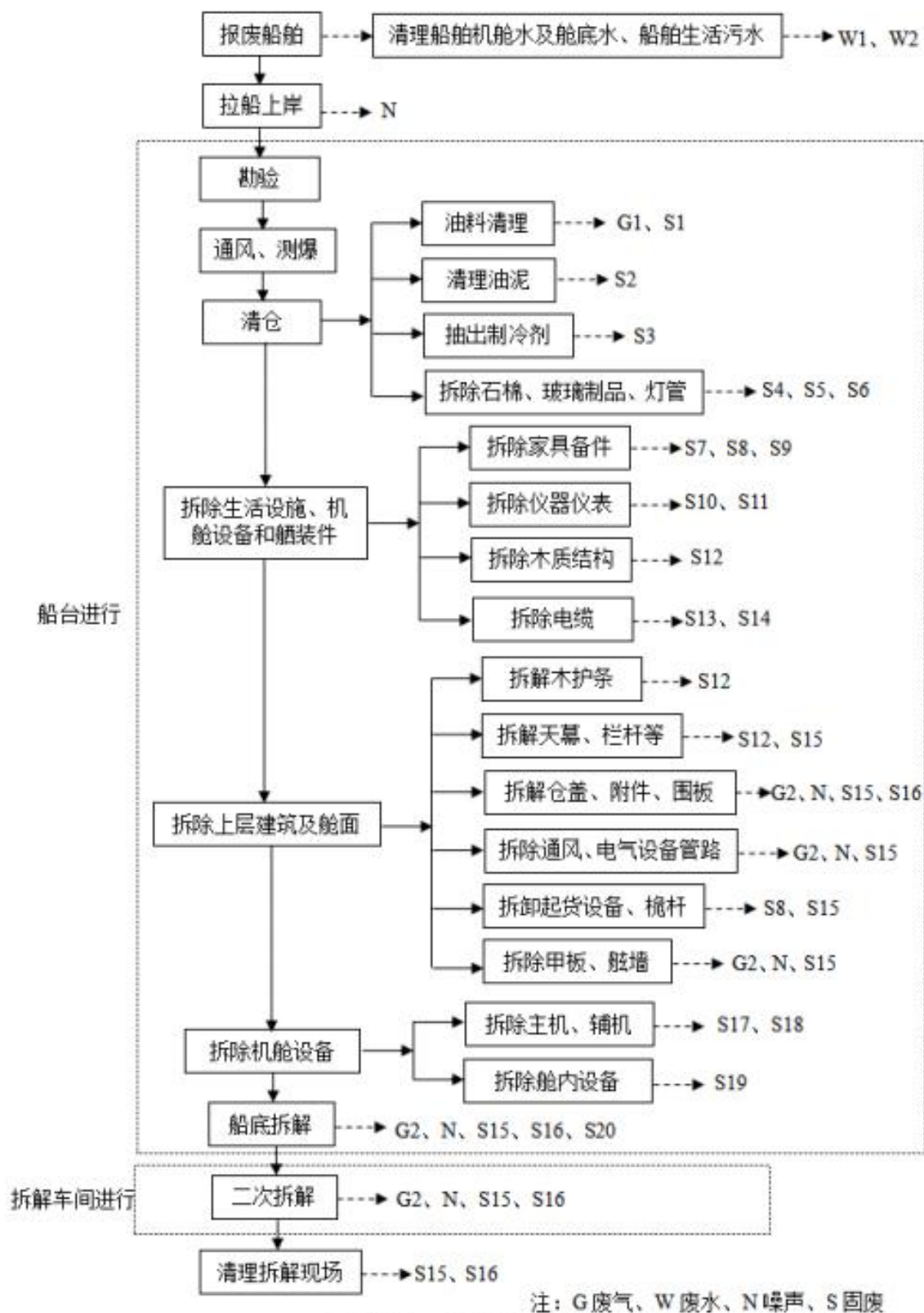
图 3.4-3 船舶拆解生产工艺流程图
