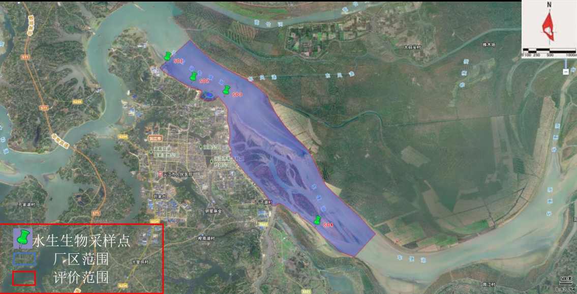
水生生物采样点布置示意图
