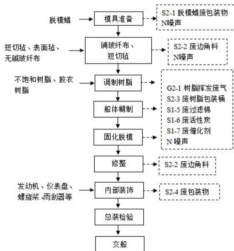
图 3.4-2 非金属（玻璃钢）船舶生产工艺流程图
