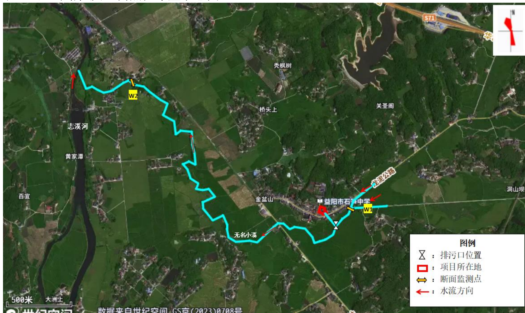
附图 10：入河路径及监测点位布置示意图
