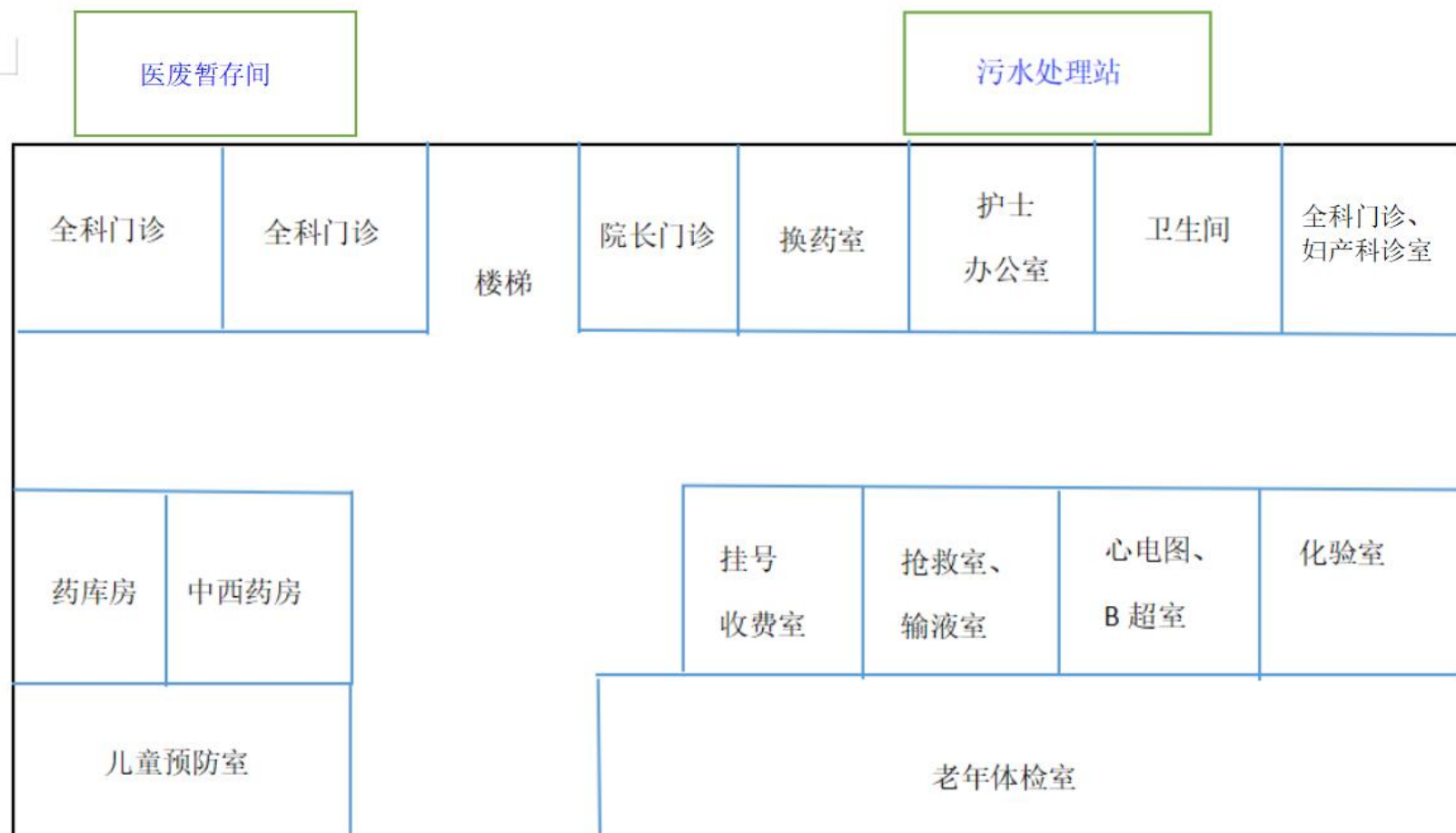
附图 3-1：门诊住院楼一层平面布置图
