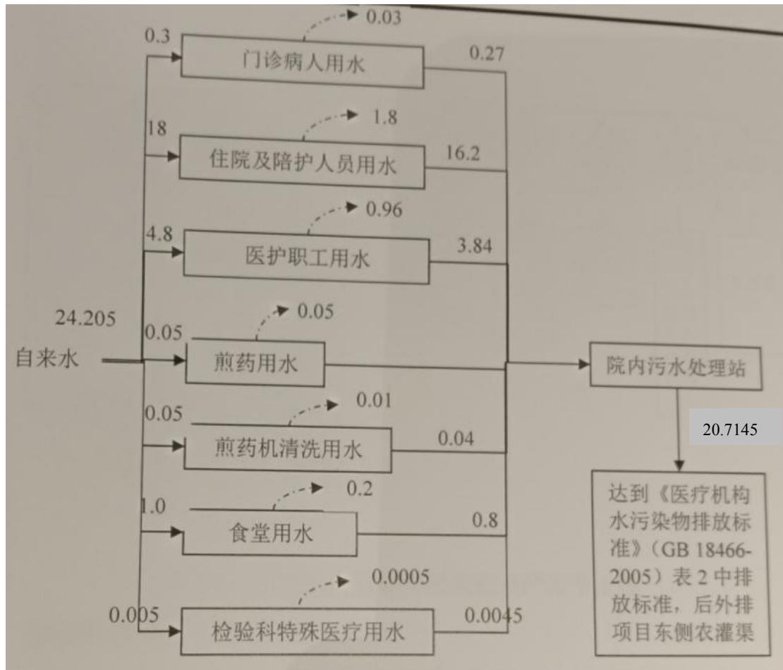
图 2.1-1 水平衡图
