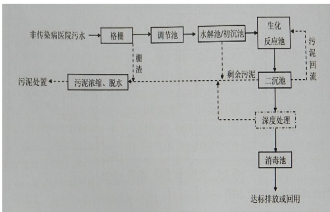
图 8.1-1. 污水处理工艺流程图
