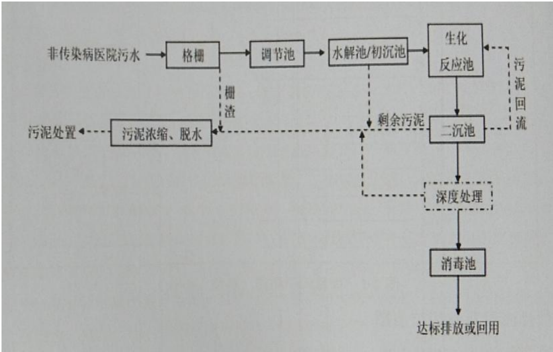
图 2.1-1.工艺流程图
