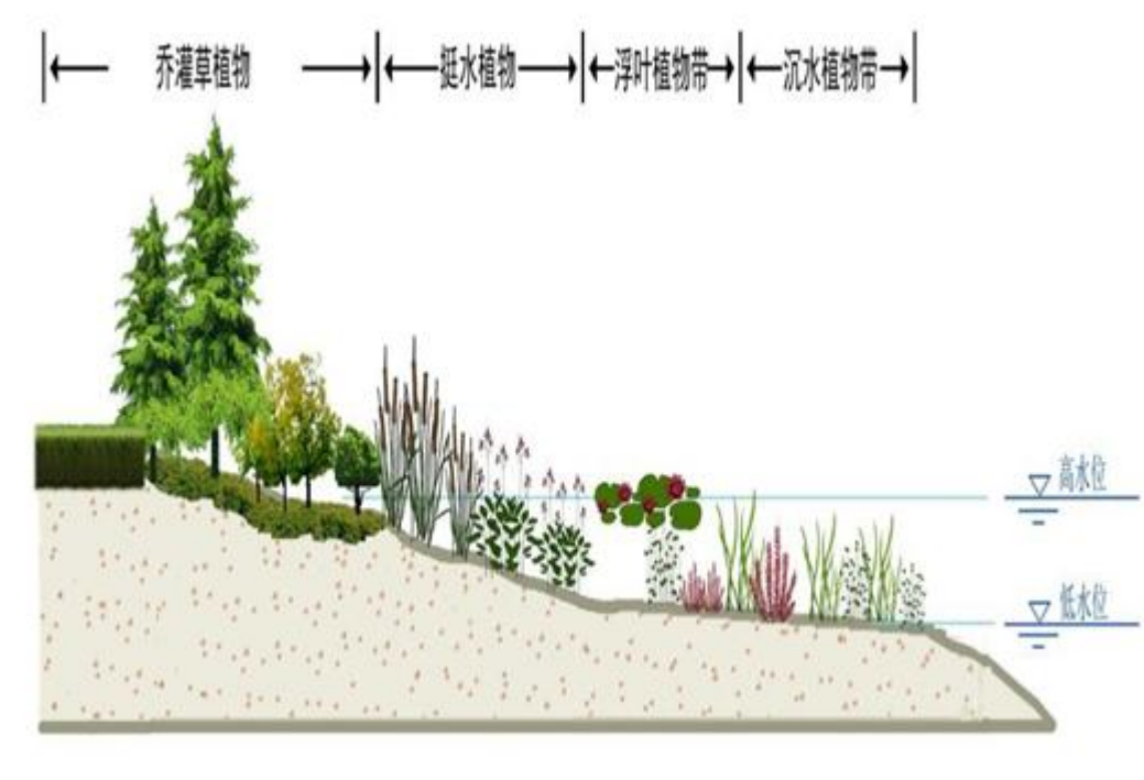
图 3.3-2 水生植被带构建示意图
