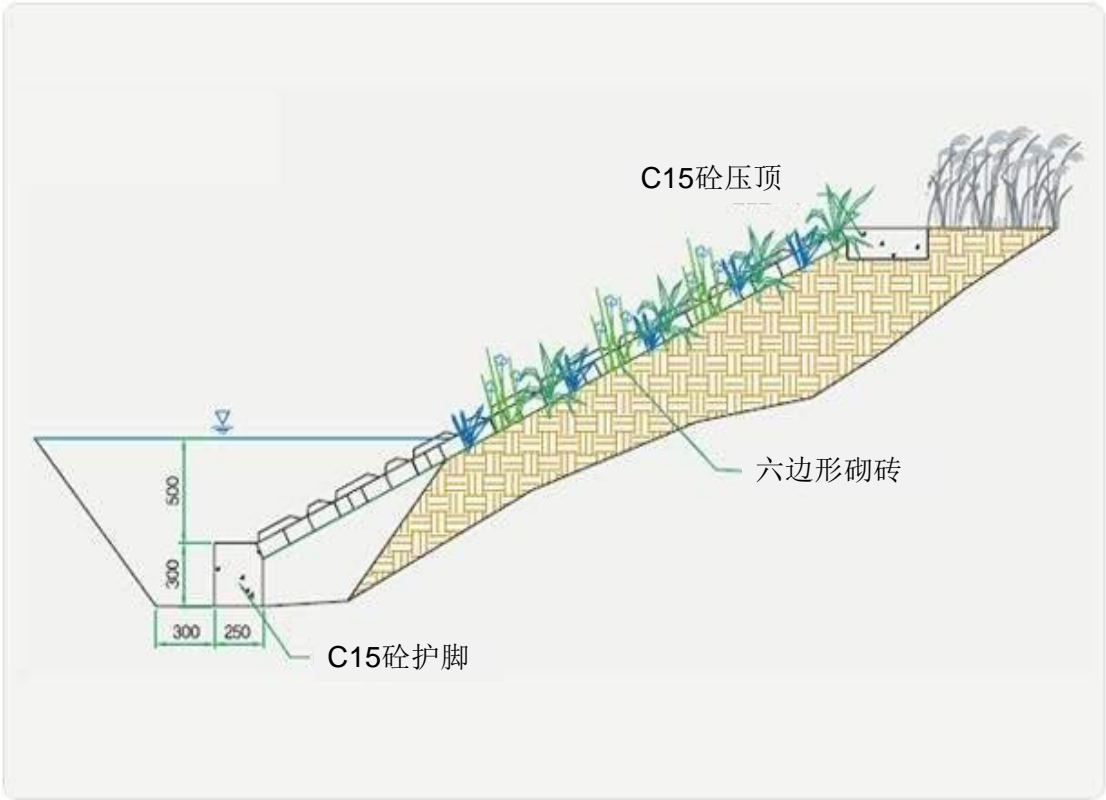
图3.3-2 生态护岸工程设计截面图
