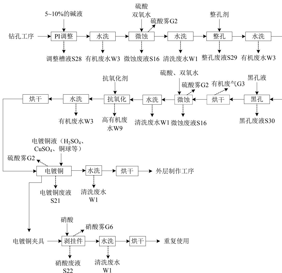
图 1.6.2-28：化学黑孔和电镀铜联合孔金属化工艺流程及产污节点图
