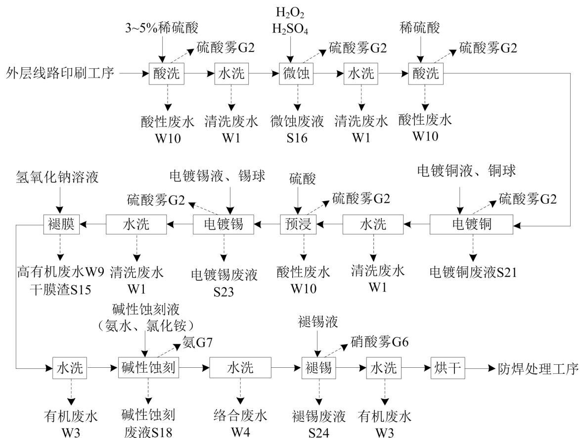
图 1.6.2-16: 正片制作工艺流程及产污节点图
