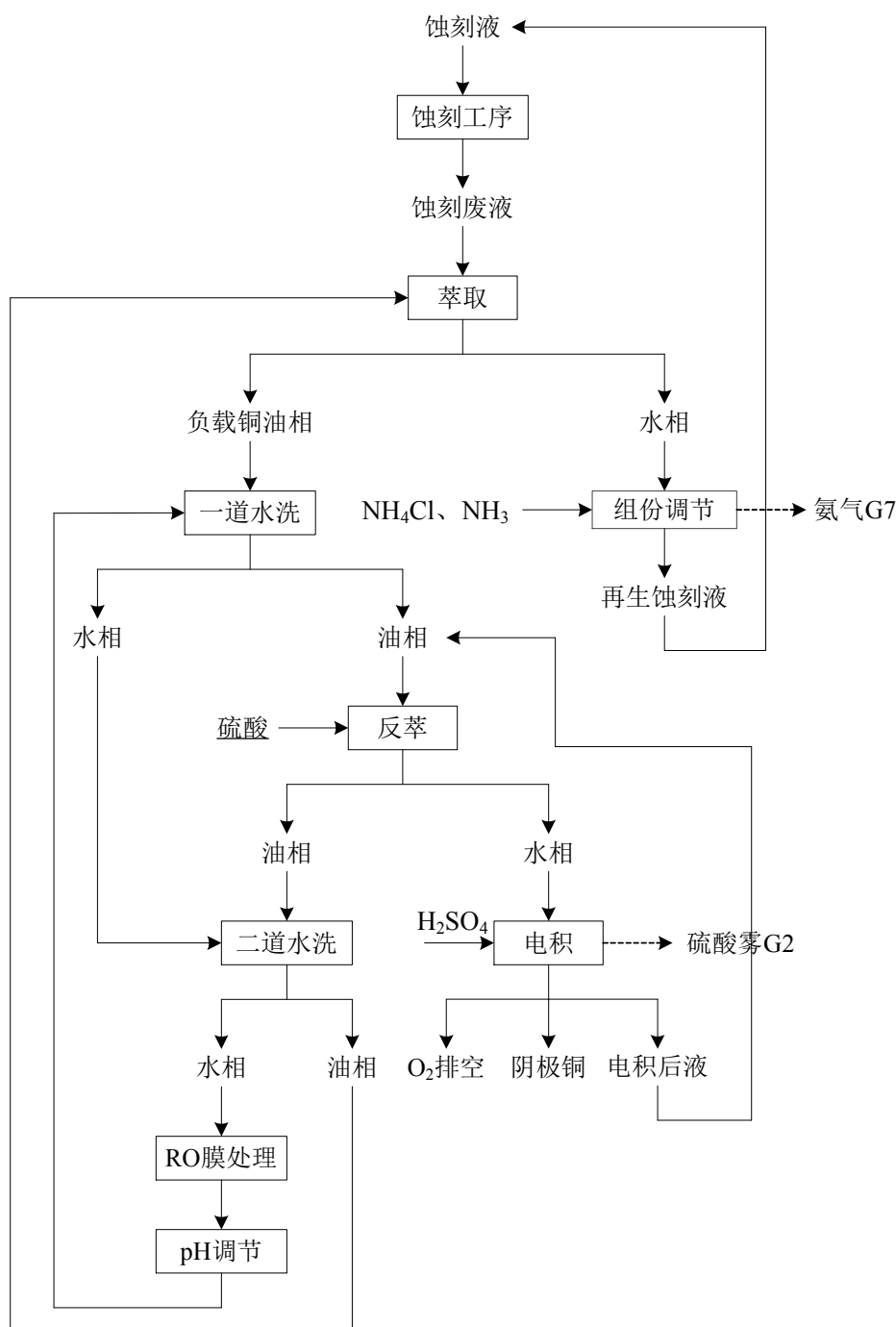
图 1.6.3-3: 碱性蚀刻废液循环系统工艺流程及产污节点图
