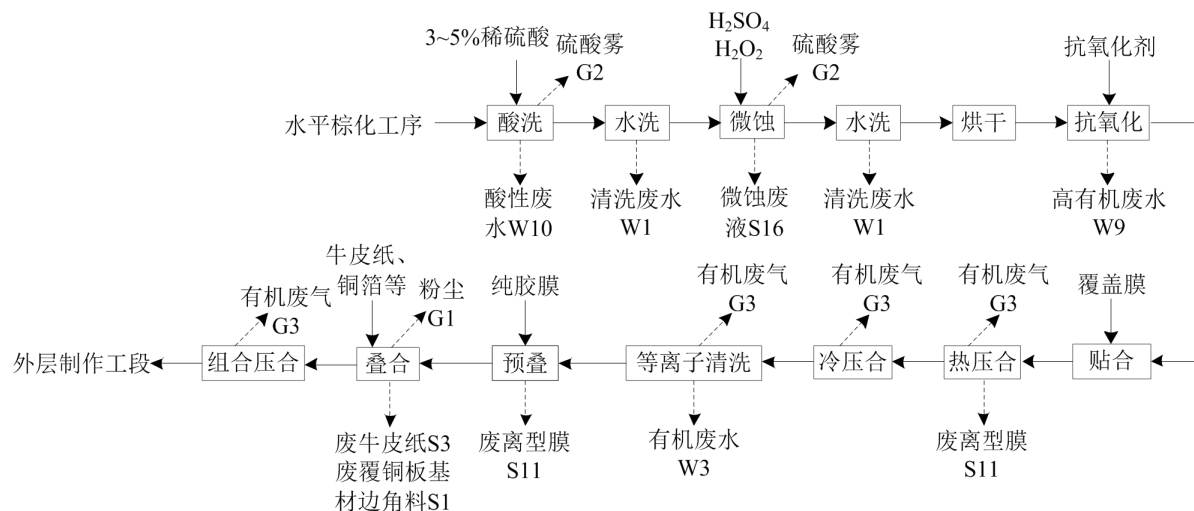
图 1.6.2-27：子板压合工序工艺流程及产污节点图
