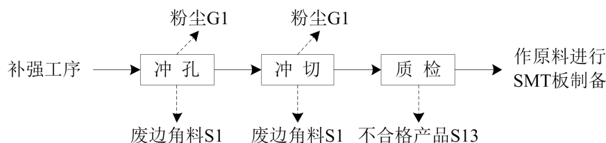
图 1.6.2-33: 成品成型工段工艺流程及产污节点图
