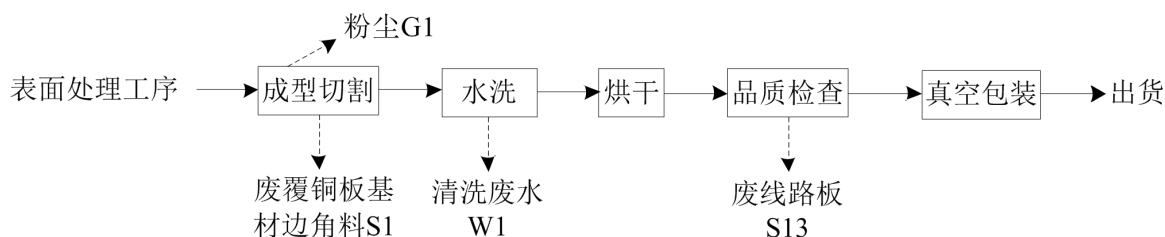
图 1.6.2-23: 成品成型工序工艺流程及产污节点图
