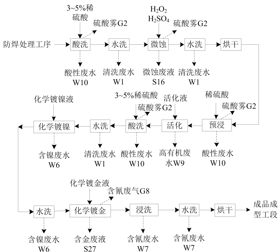
图 1.6.2-22：化学镀镍金操作单元生产工艺流程及产污节点图
