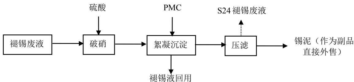
图 1.6.3-6: 褪锡废液回收工艺流程及产排污节点图
