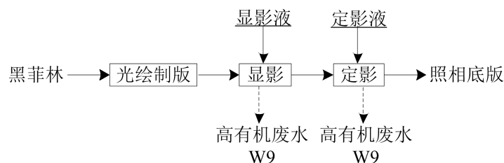
图 1.6.2-1：照相底版制作工序工艺流程及产污节点图
