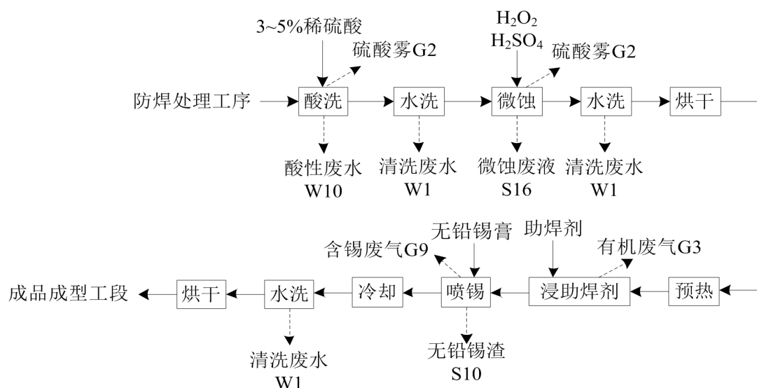
图 1.6.2-19：无铅喷锡（热风整平）工艺流程及产污节点图
