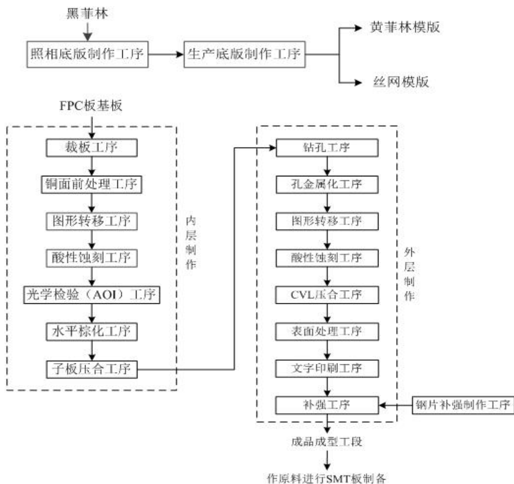
图 4-2 FPC 板生产工艺流程图
