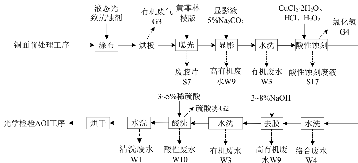
图 1.6.2-7：图形转移、酸性蚀刻工艺流程及产污节点图
