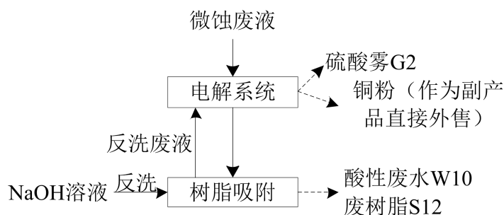
图 1.6.3-4：微蚀废液铜回收工艺流程及产排污节点图
