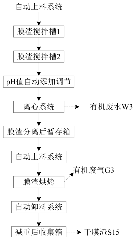
图 1.6.3-7：干膜渣减重工艺流程及产排污节点图
