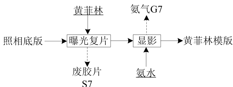
图 1.6.2-2：黄菲林模版制作工艺及产污节点图
