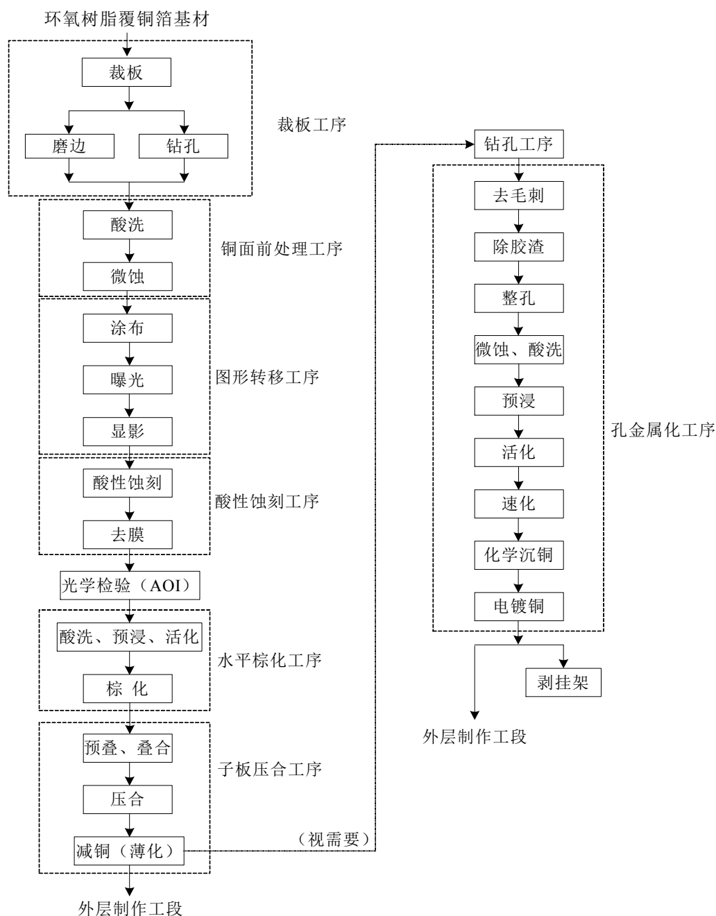
图 1.6.2-4：内层制作工艺流程简图
