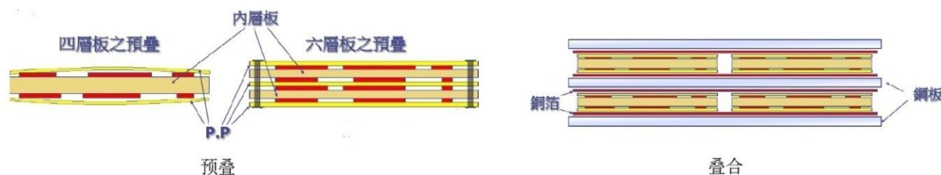
图 1.6.2-9 预叠和叠合结构示意图
