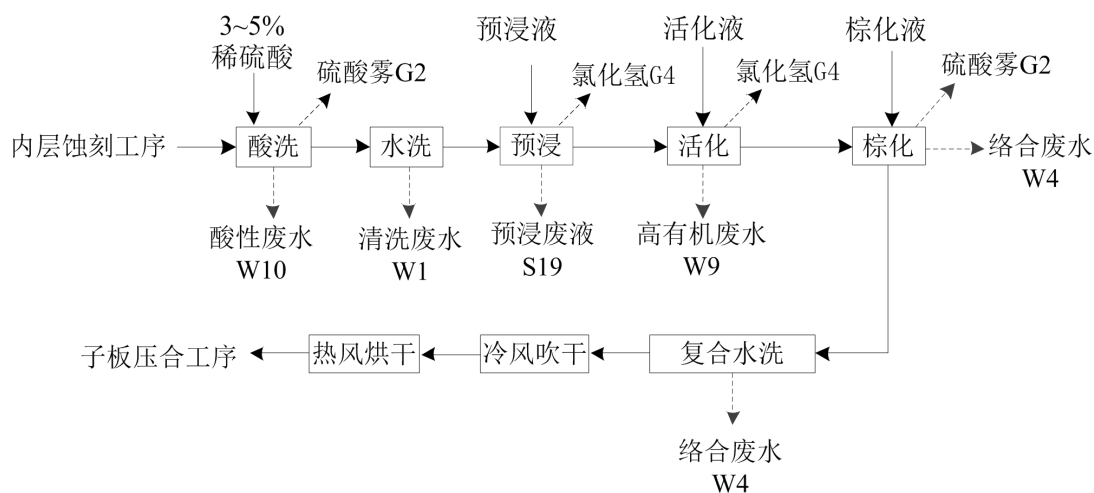
图 1.6.2-8 水平棕化工序工艺流程及产污节点图
