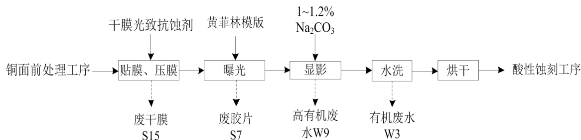
图 1.6.2-25: 图形转移工序工艺流程及产污节点图
