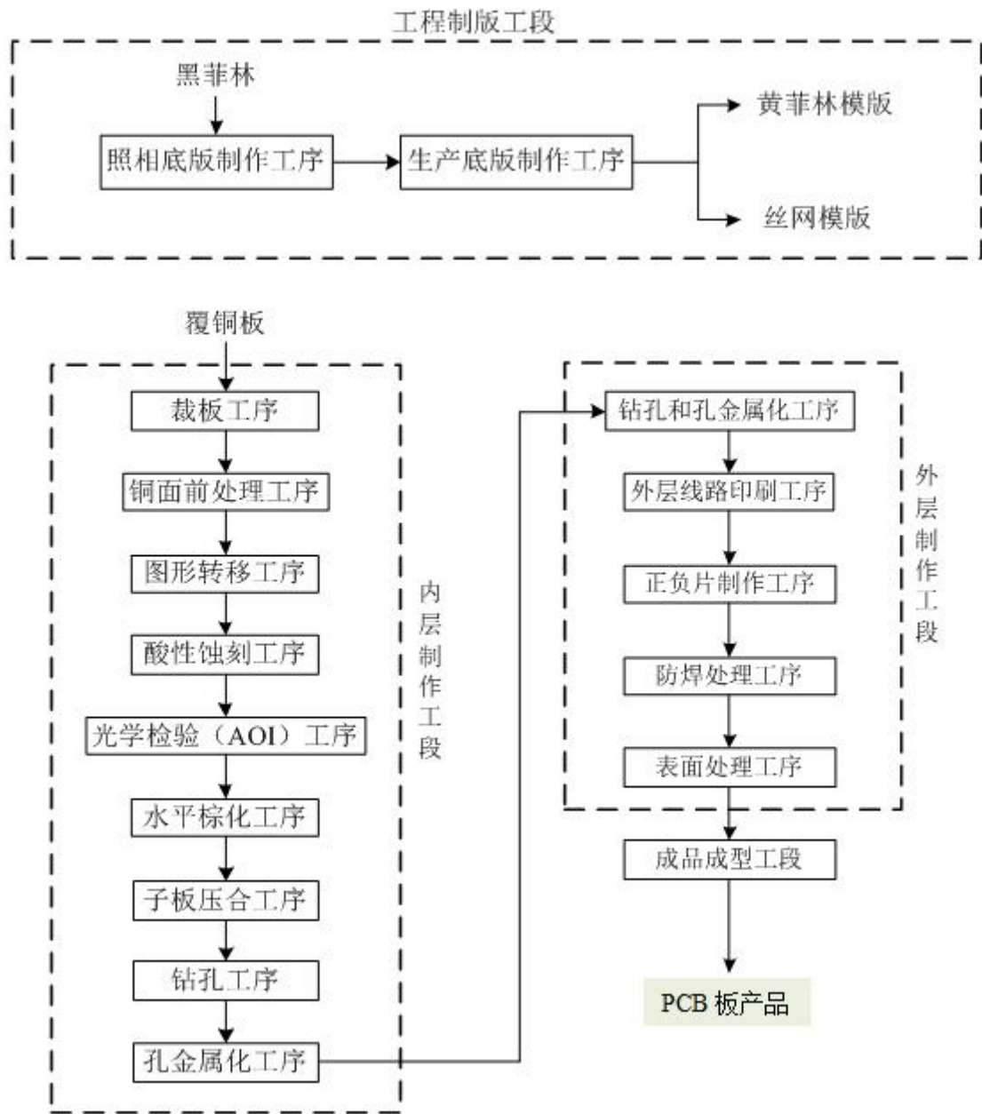
图 4-1 PCB 板生产工艺流程图
