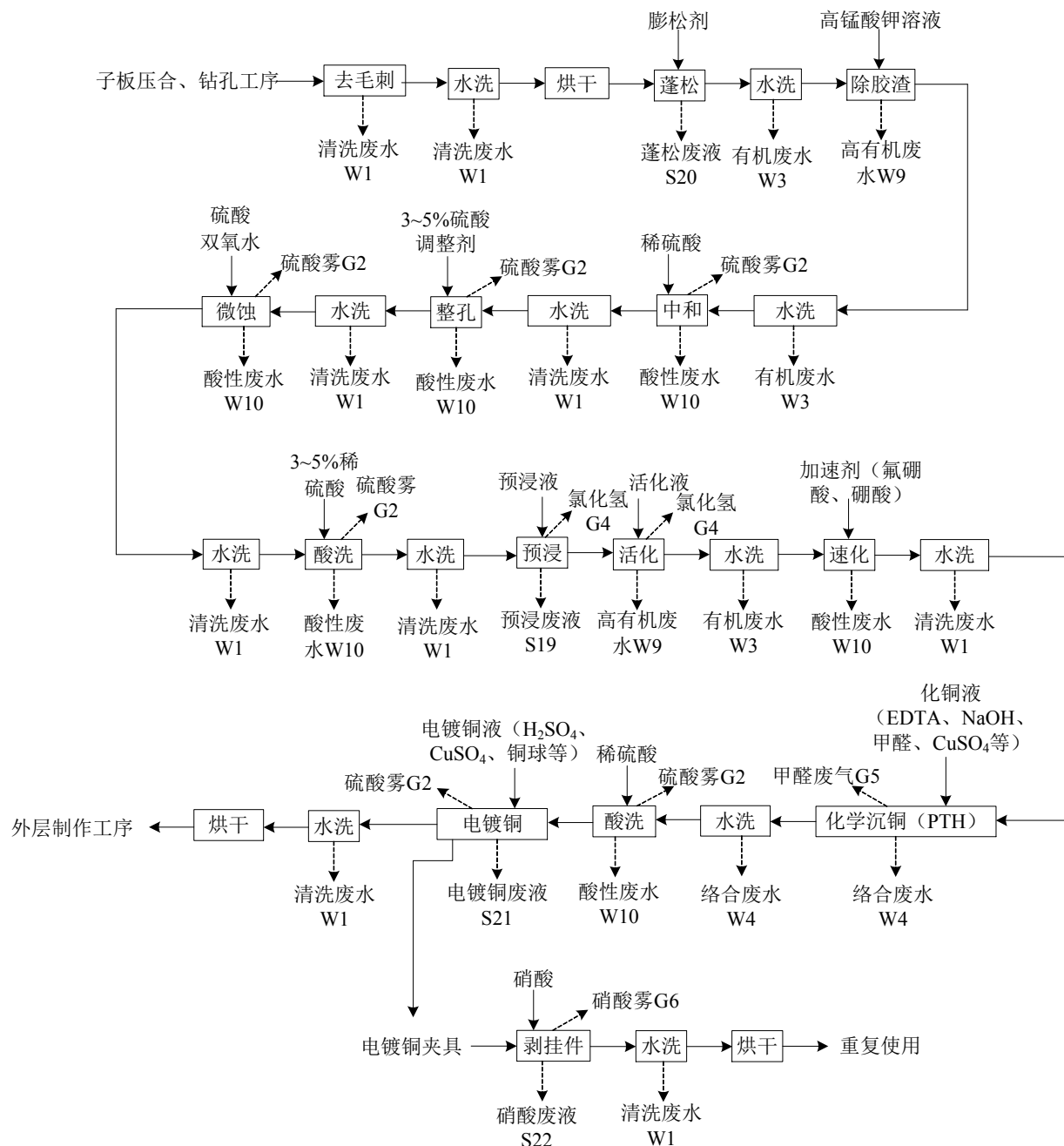
图 1.6.2-12: 孔金属化工序工艺流程及产污节点图
