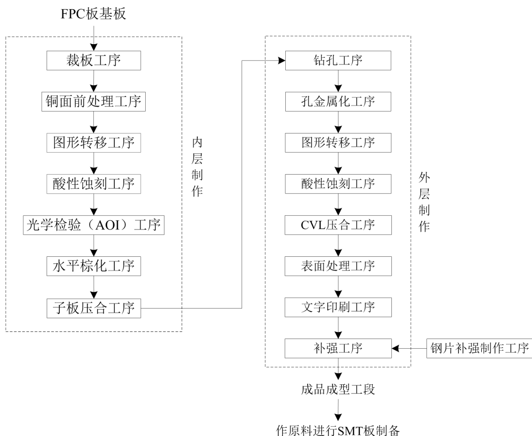
图 1.6.1-2 FPC 多层板生产工艺流程图
