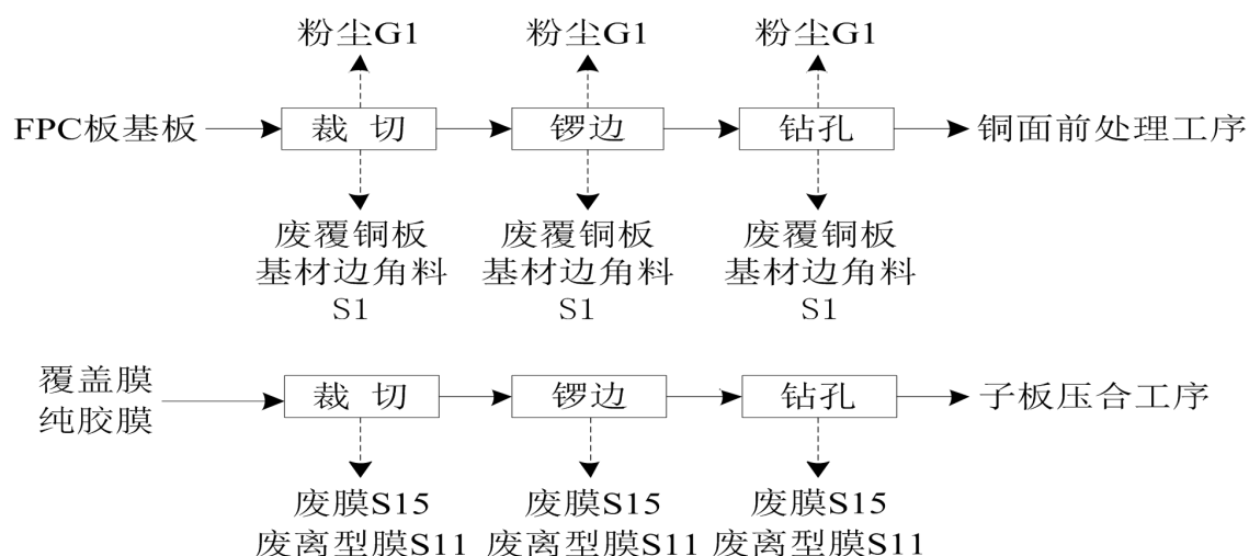
图 1.6.2-24：裁板工序工艺流程及产污节点图
