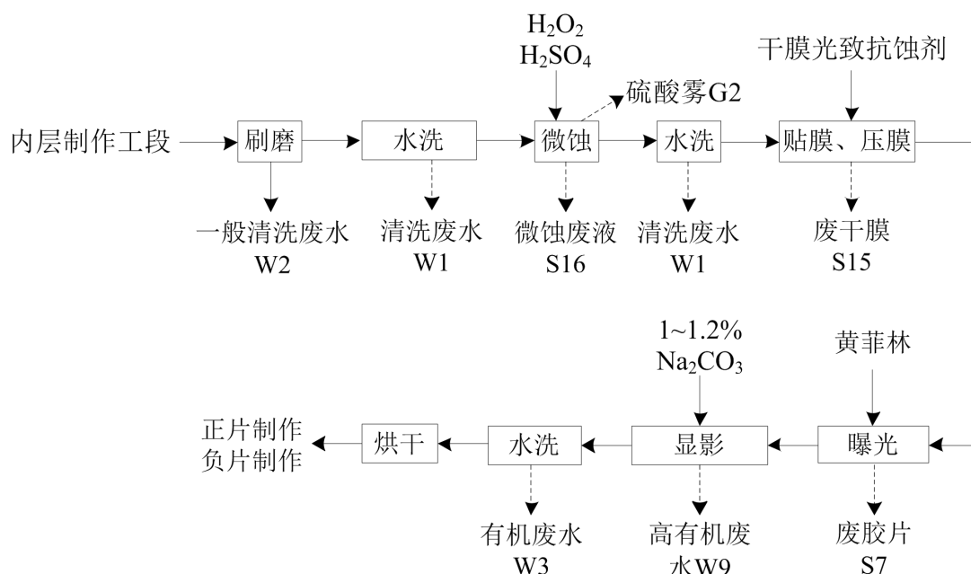
图 1.6.2-14：外层线路印刷工序工艺流程及产污节点图
