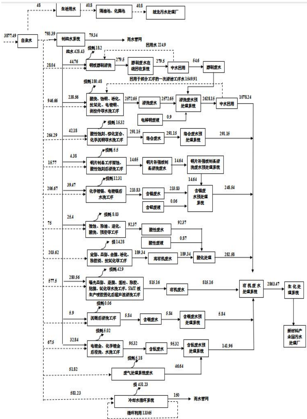
图 1.5-1 水平衡图 (单位 m 3 /d)
