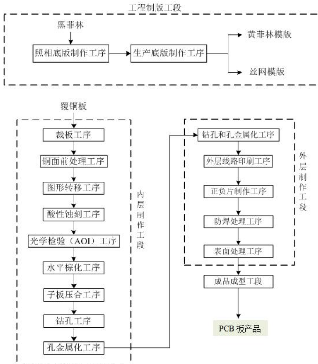
图 1.6.1-1 PCB 多层板生产工艺流程图
