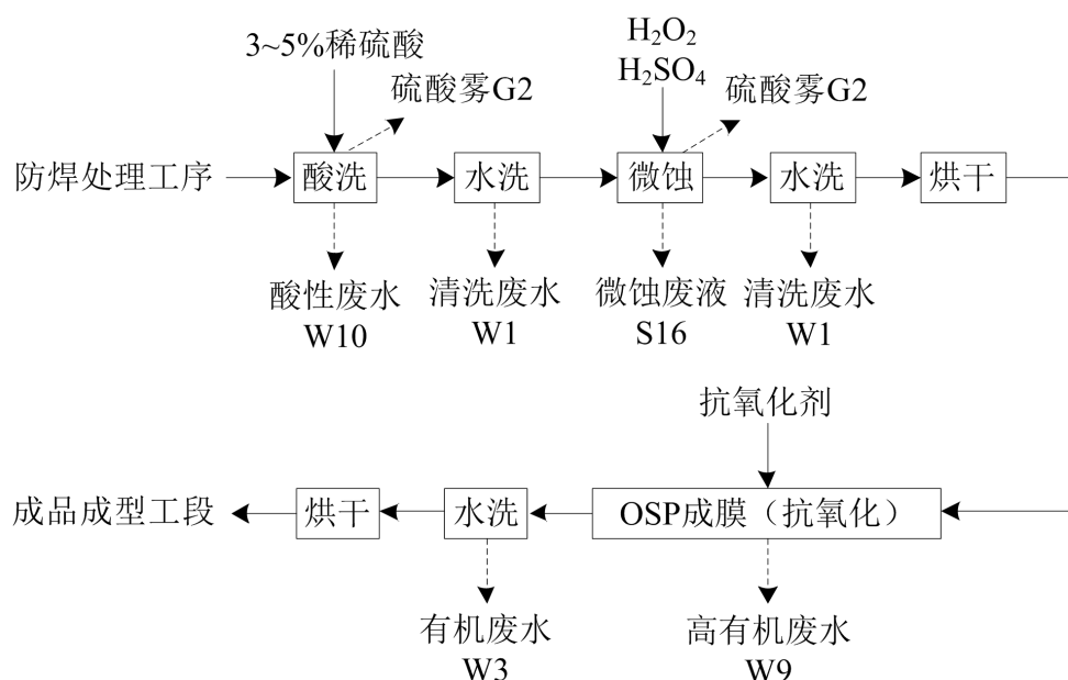
图 1.6.2-18: OSP（抗氧化）表面处理操作单元工艺流程及产污节点图
