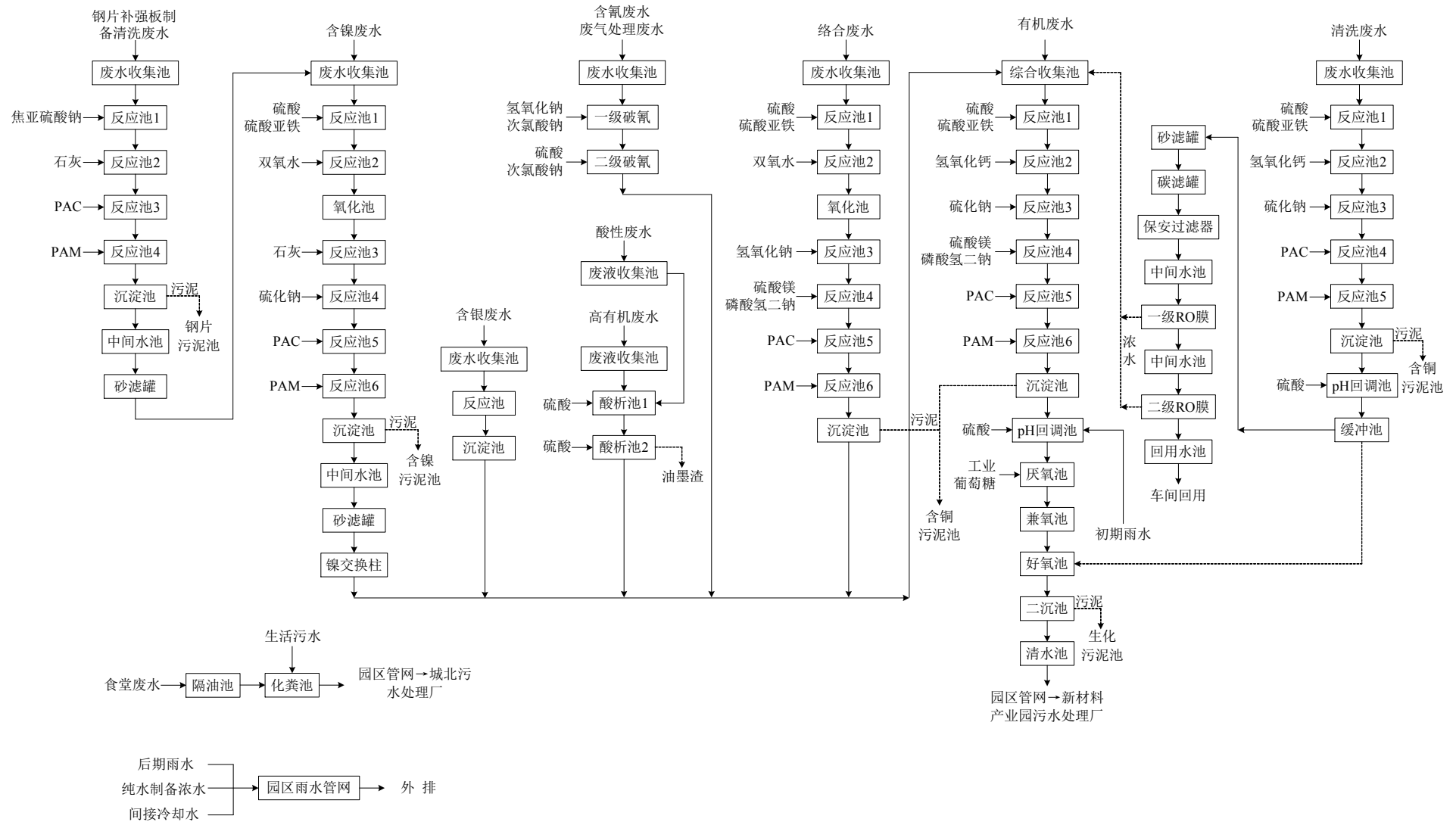
图 1.7.2-1: 废水处理总体方案及走向示意图
