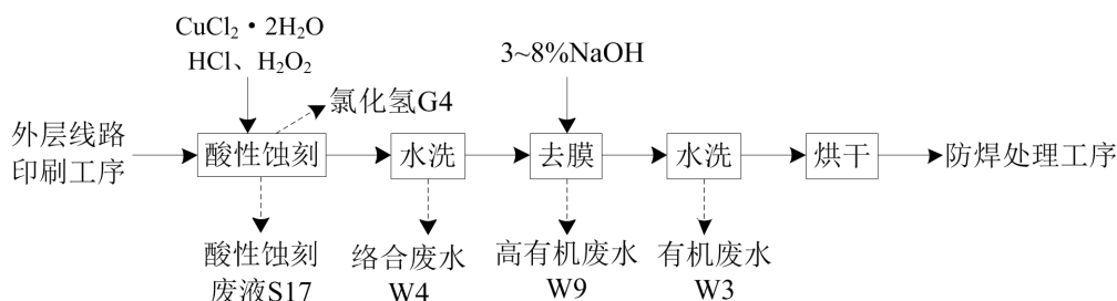
图 1.6.2-15：负片制作工艺流程及产污节点图
