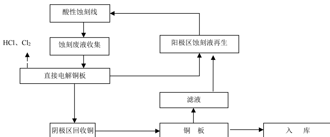
图 1.6.3-2：酸性蚀刻废液循环系统工艺流程及产污节点图
