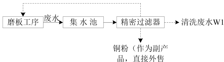
图 1.6.3-1：刷磨废水在线回收铜粉工艺流程及产污节点图
