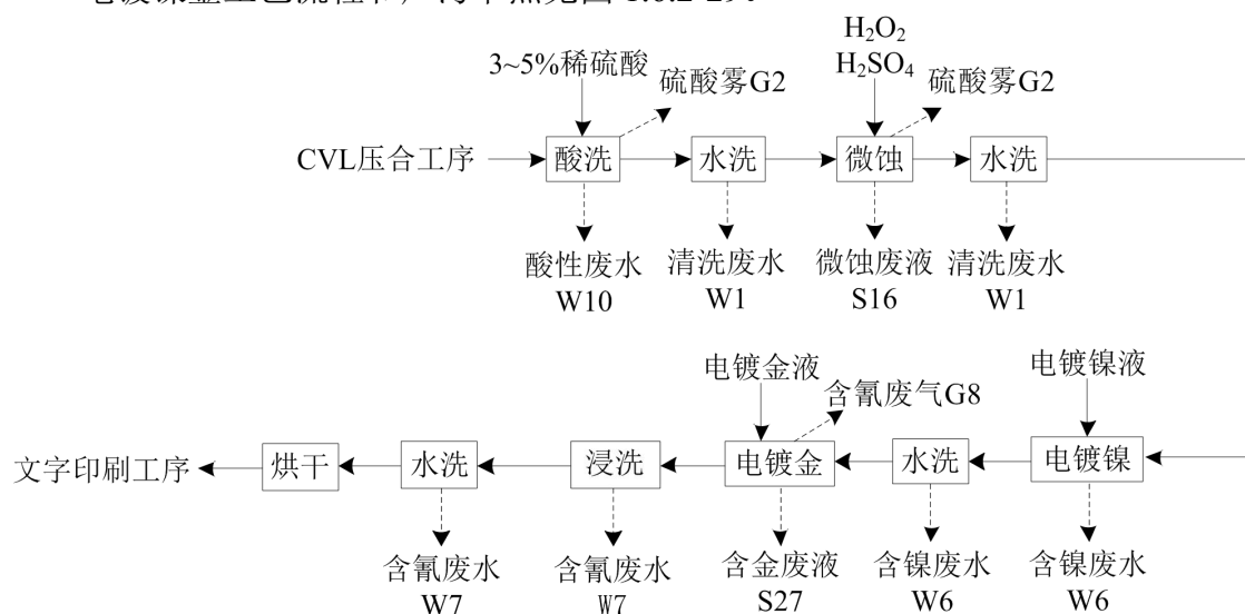
图 1.6.2-29：电镀镍金工艺流程及产污节点图
