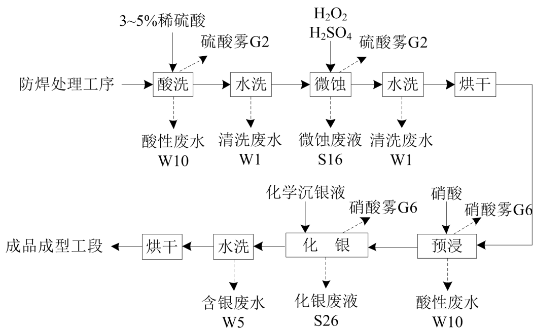
图 1.6.2-20: 化学沉银操作单元流程及产污节点图
