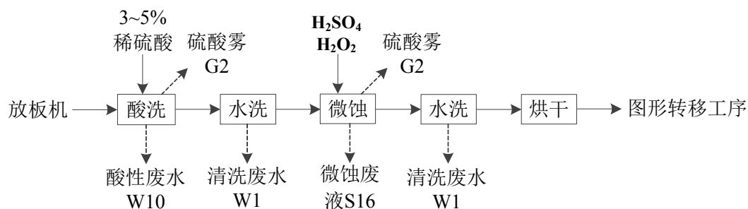
图 1.6.2-6: 铜面前处理工序工艺流程及产污节点图
