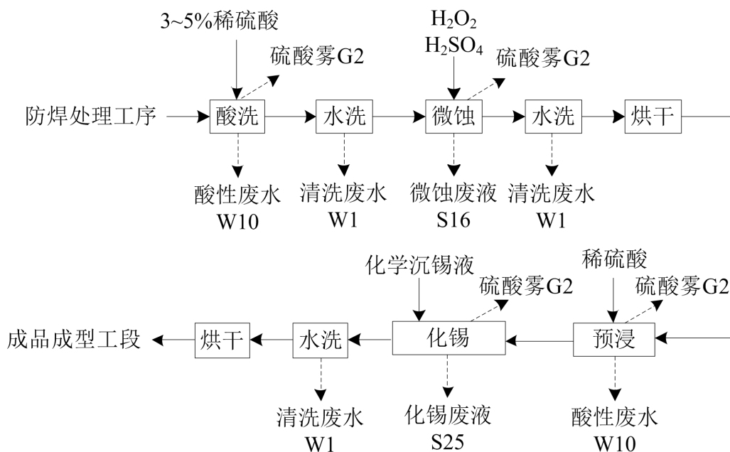
图 1.6.2-21: 化学沉锡操作单元工艺流程及产污节点图
