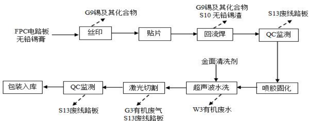
图 4-3 表面组装（SMT）工艺流程图
