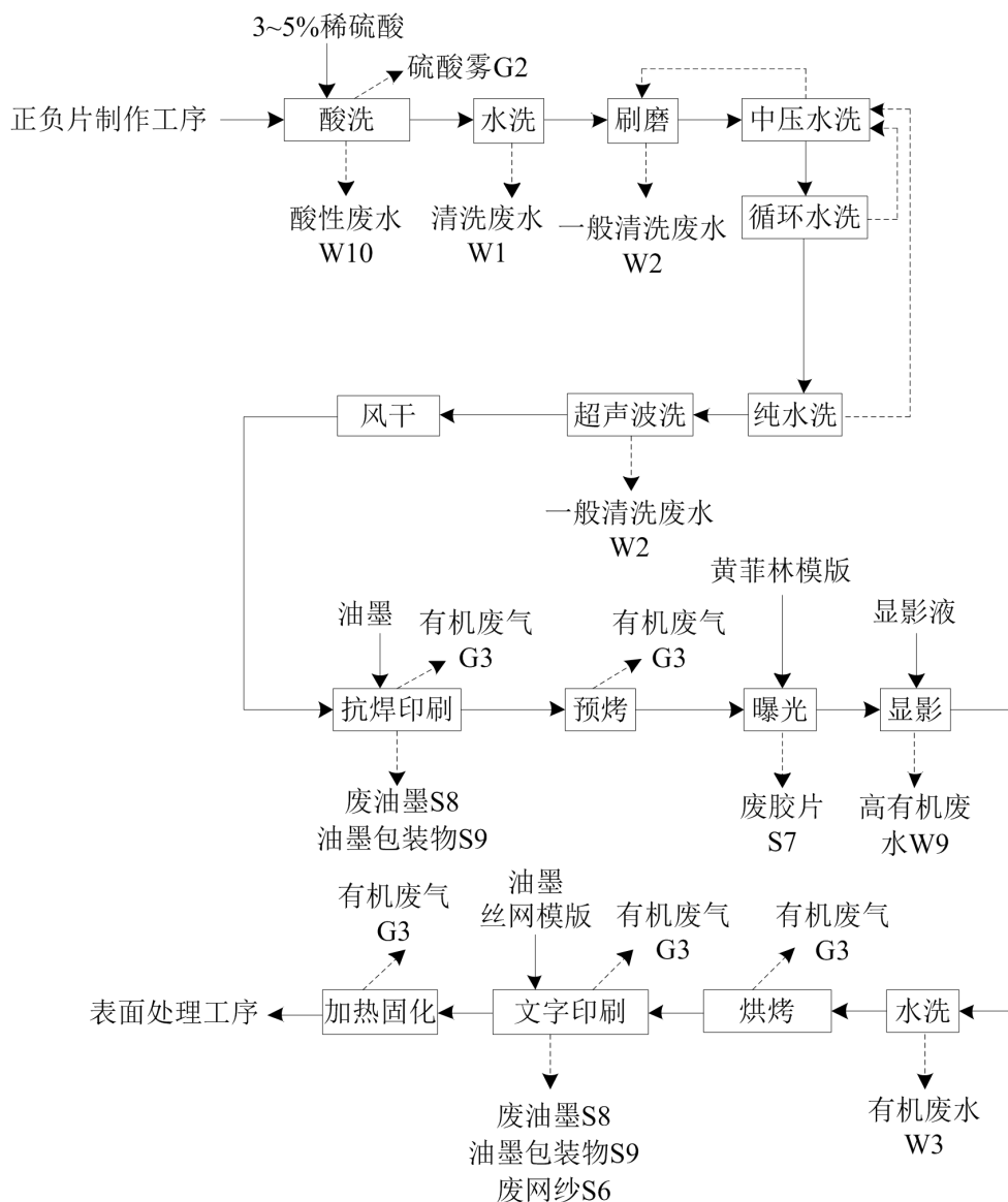
图 1.6.2-17: 防焊处理工序生产工艺流程及产污节点图
