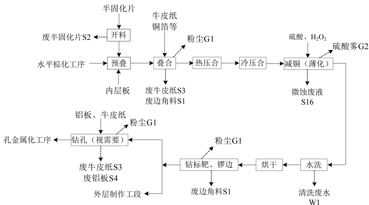
图 1.6.2-11: 子板压合、钻孔工序工艺流程及产污节点图
