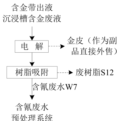
图 1.6.3-5: 含金废液/废水金回收系统工艺流程及产污节点图
