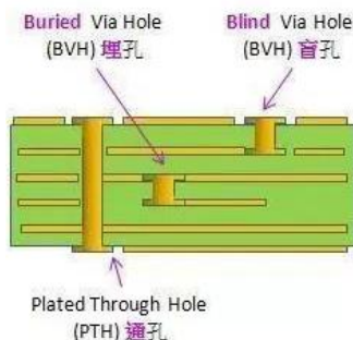
图 1.6.2-10: 埋孔结构示意图
