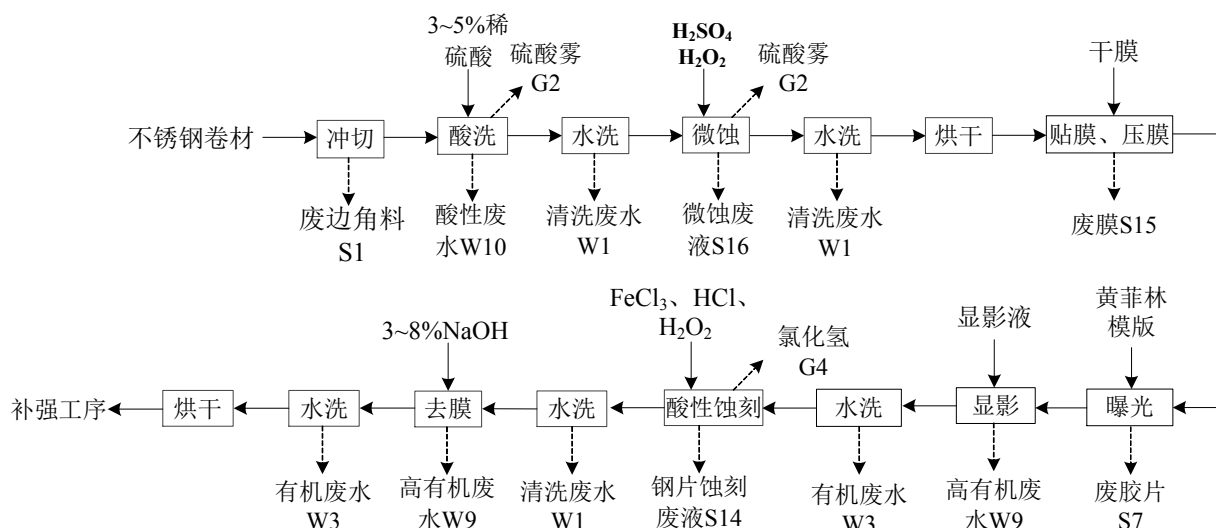
图 1.6.2-31: 钢片补强板制备工段工艺流程及产污节点图
