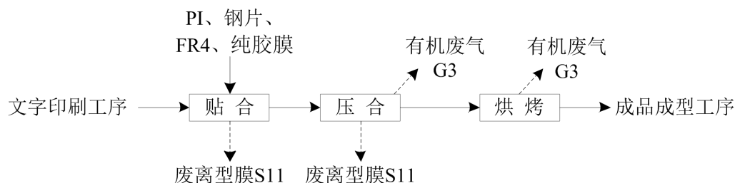
图 1.6.2-32: 补强工艺流程及产污节点图
