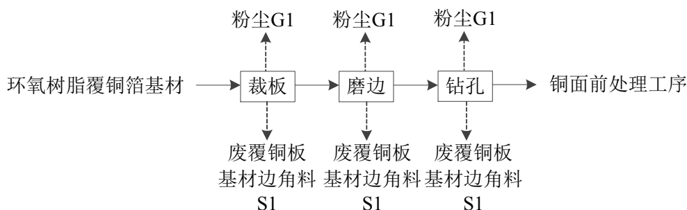
图 1.6.2-5: 裁板工序工艺流程及产污节点图 图例：G—废气、S—固废
