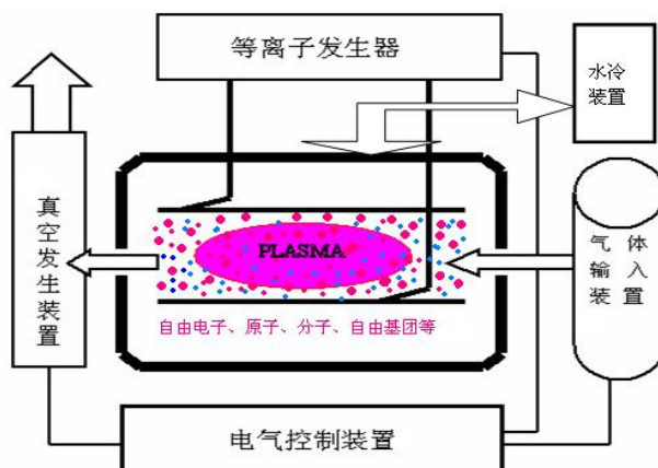
图 1.6.2-26：等离子清洗操作单元示意图
