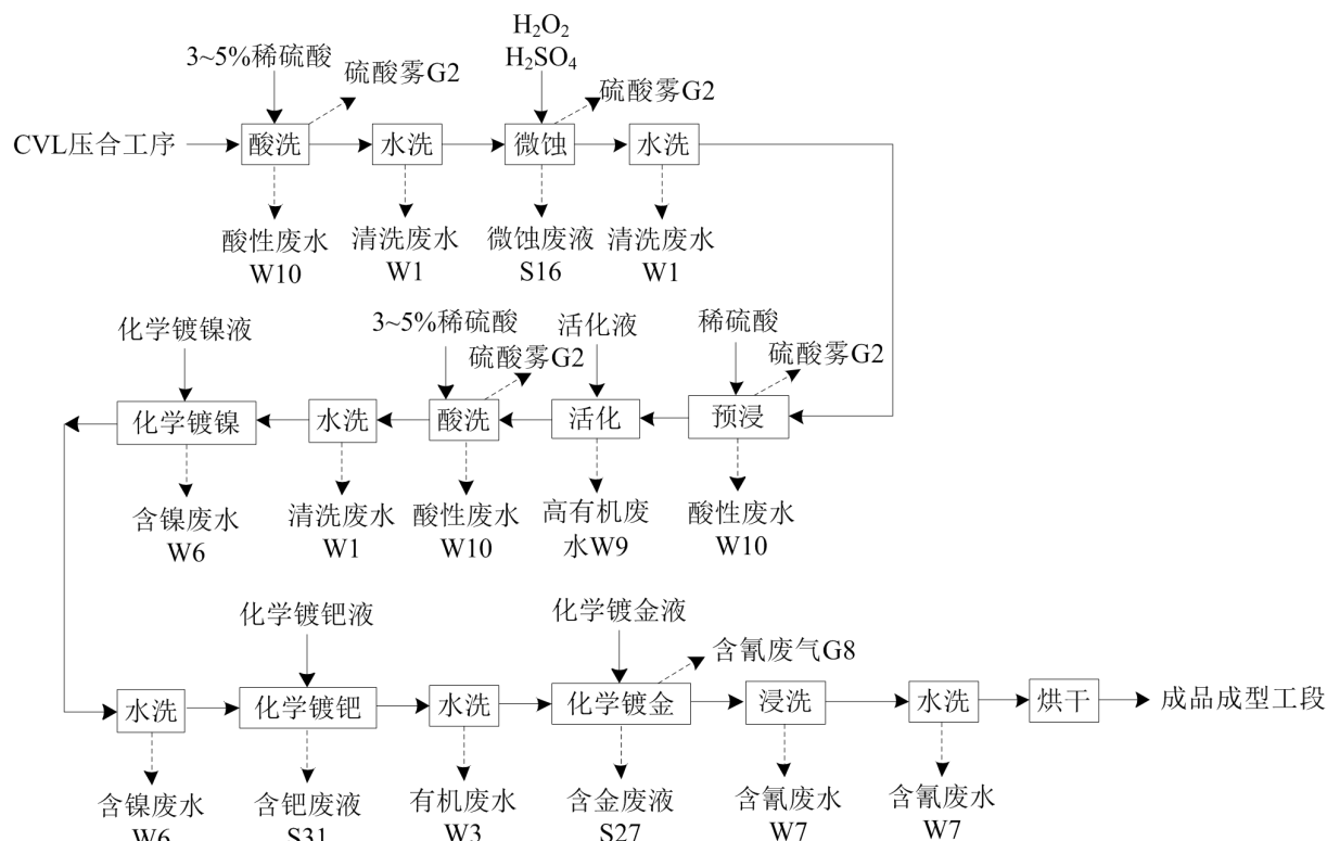
图 1.6.2-30: 化学镍钯金工艺流程及产污节点图
