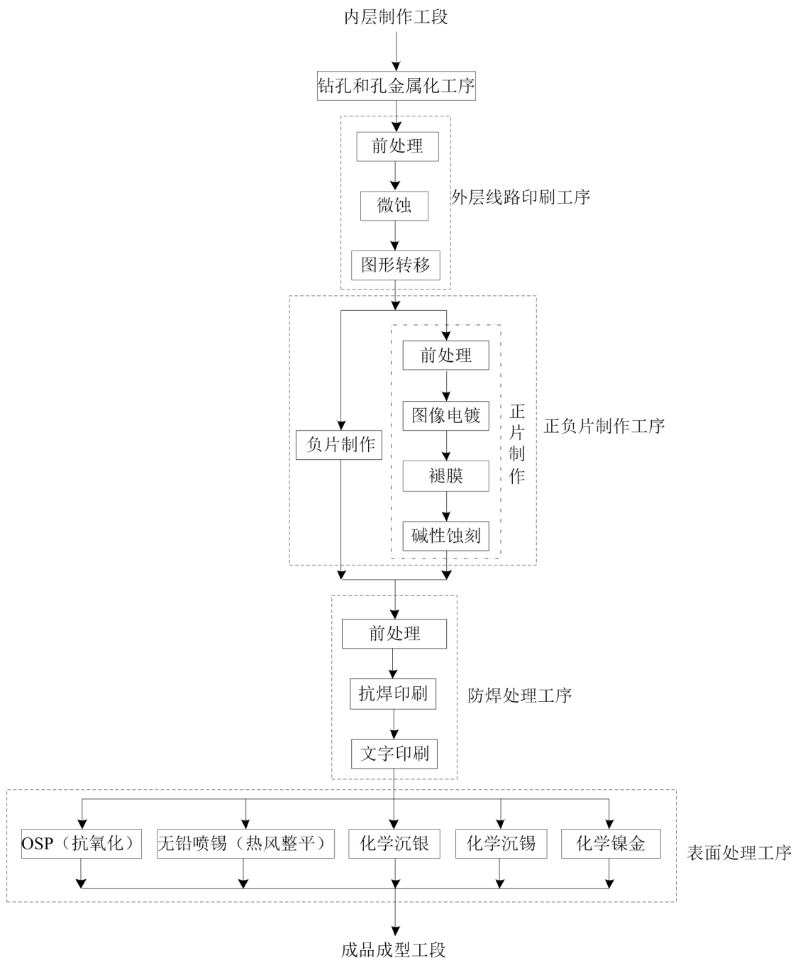
图 1.6.2-13：外层制作工段工艺流程简图
