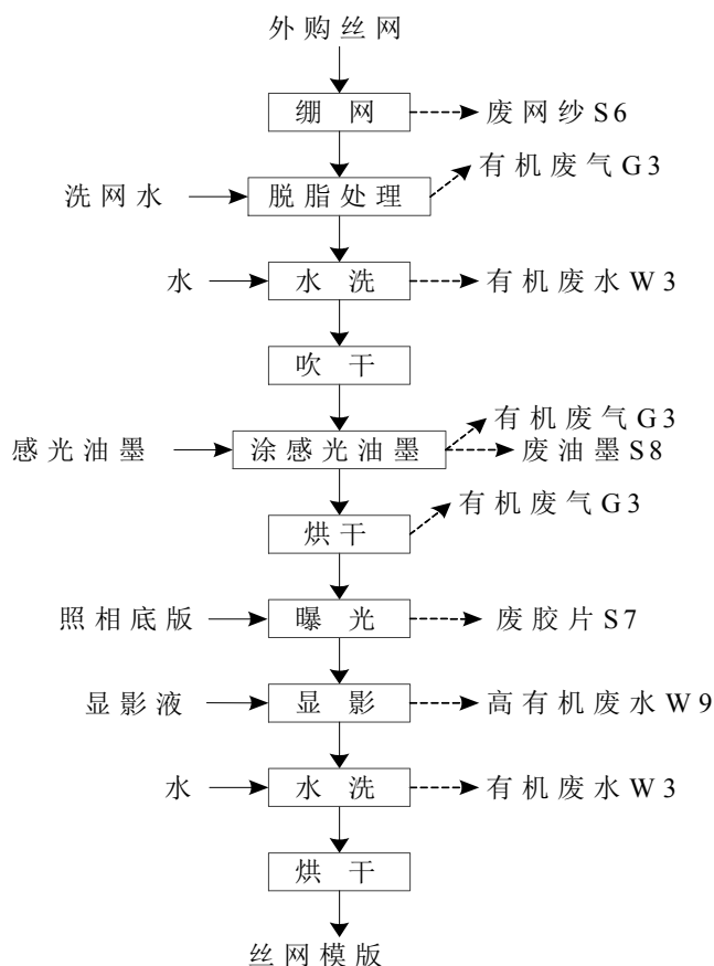
图 1.6.2-3：丝网模版制作工序工艺流程及产排污节点图
