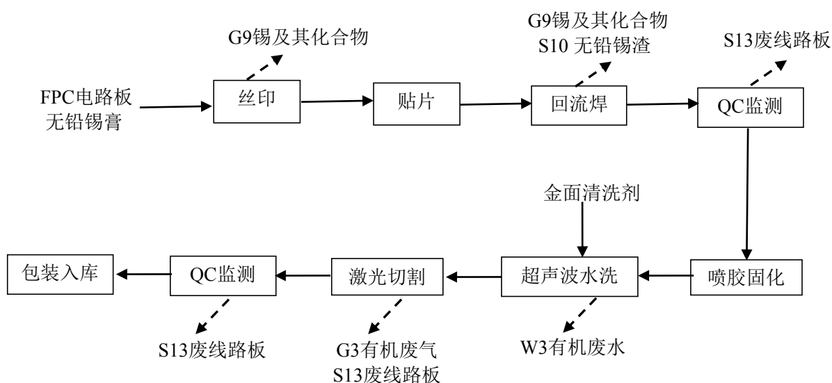
图 1.6.1-3 表面组装（SMT）工艺流程图
