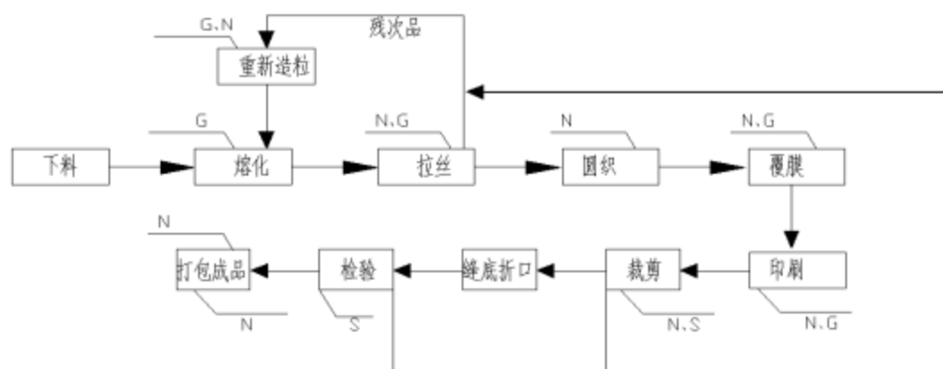
图 3.2-1 本项目生产工艺及产污节点图
