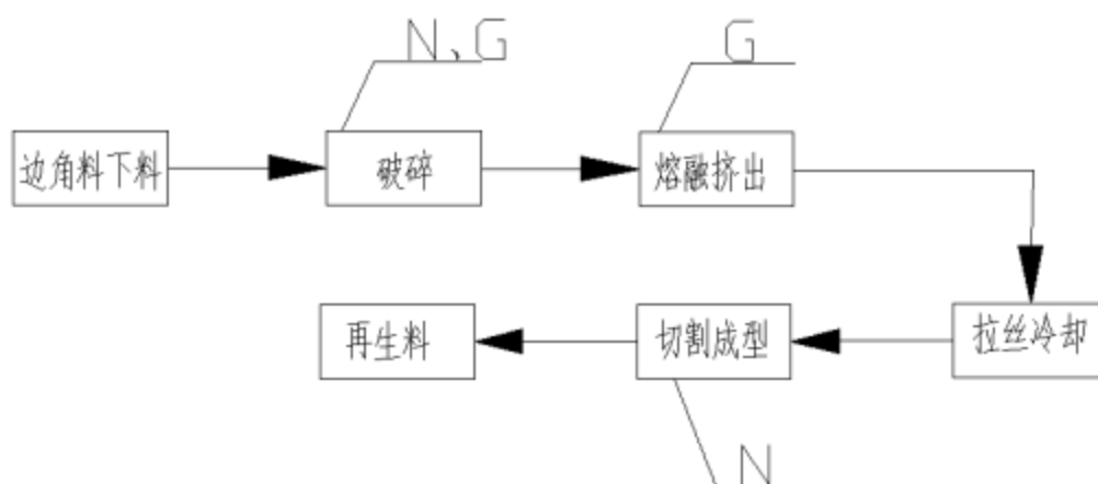
图 3.2-4 造粒工艺流程及产污节点图
