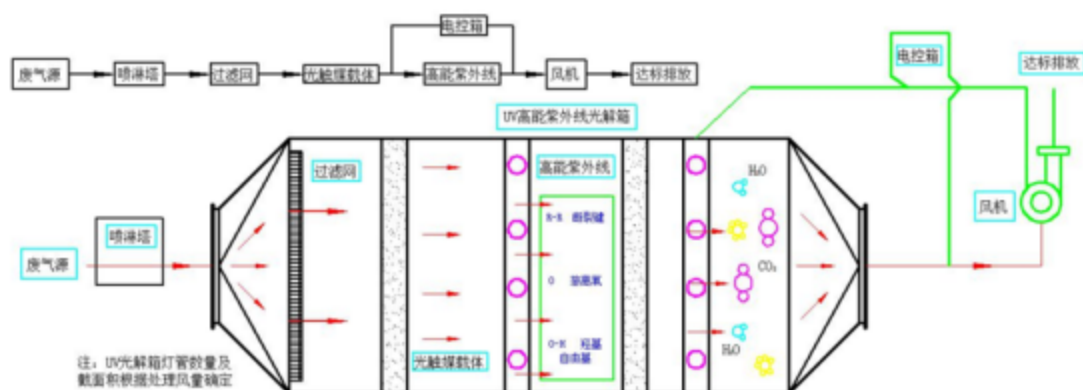
图 6.2-1 光氧催化设备工作原理示意图
