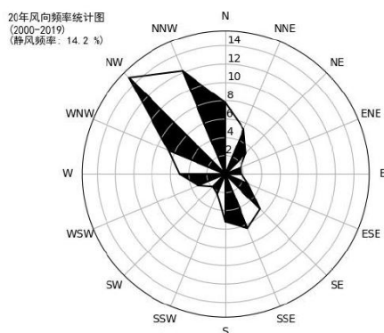
图 4.2-5 赫山风向玫瑰图(2000-2019)
