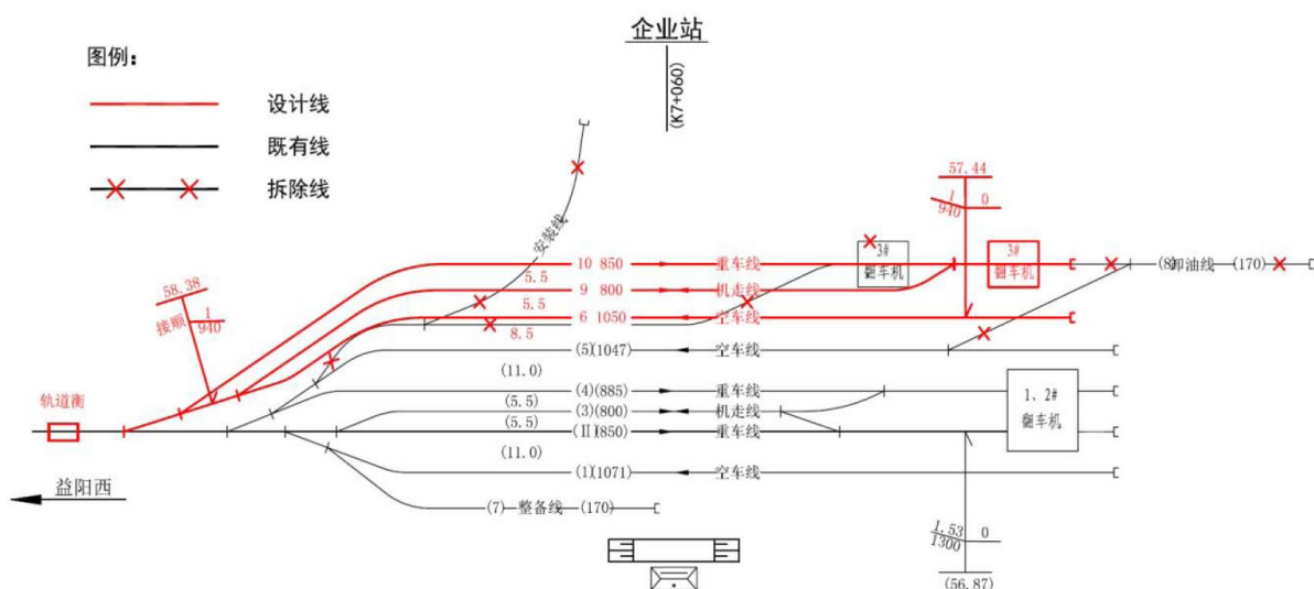
图3.3-1 改建铁路专用线示意图
