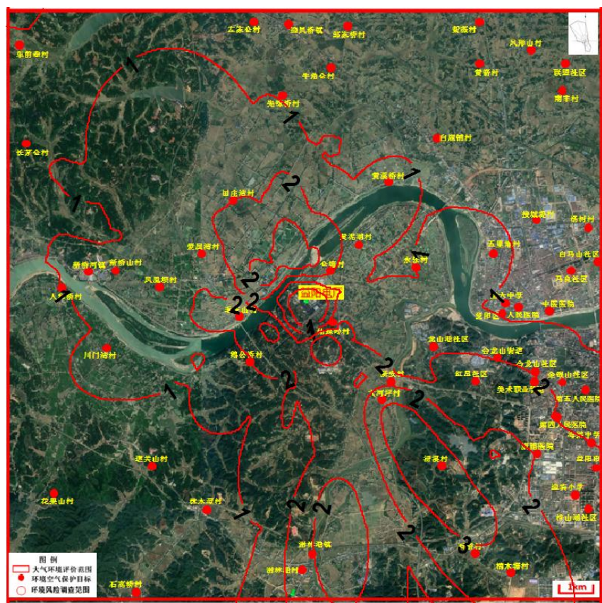
图 5.1-5 NO 2 日平均最大贡献浓度(µg/m 3 )分布图
