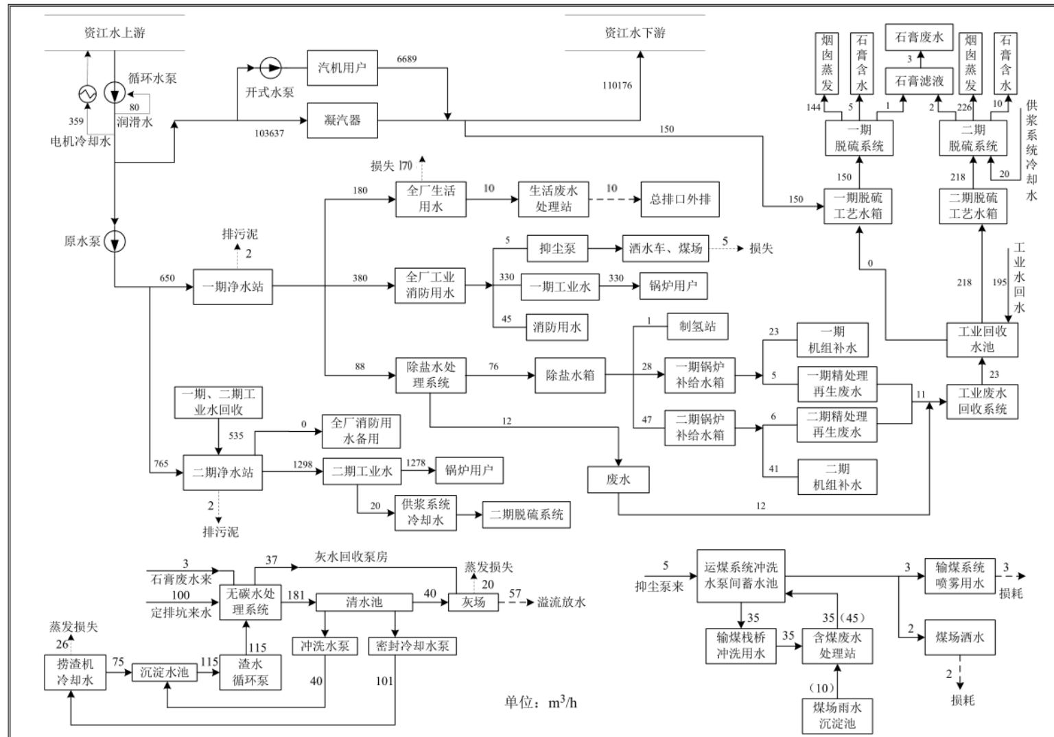
图 3.1-1 一、二期工程水量平衡示意图
