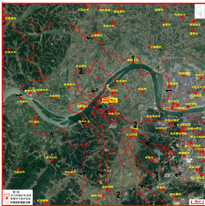
图 5.1-4 SO 2 日平均最大贡献浓度(µg/m 3 )分布图
