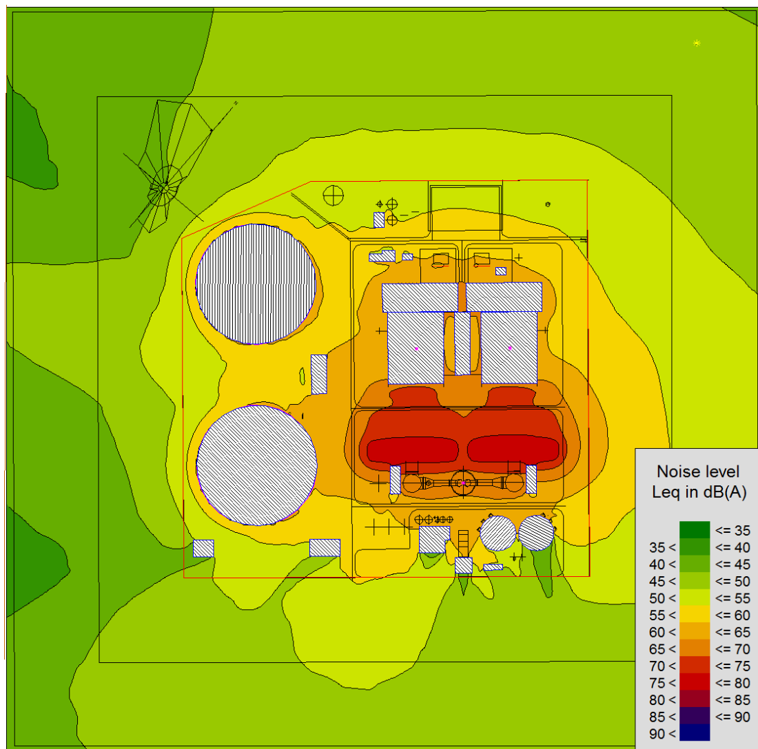
图 5.4-3 本工程锅炉排汽加消声器时噪声预测等值线图
