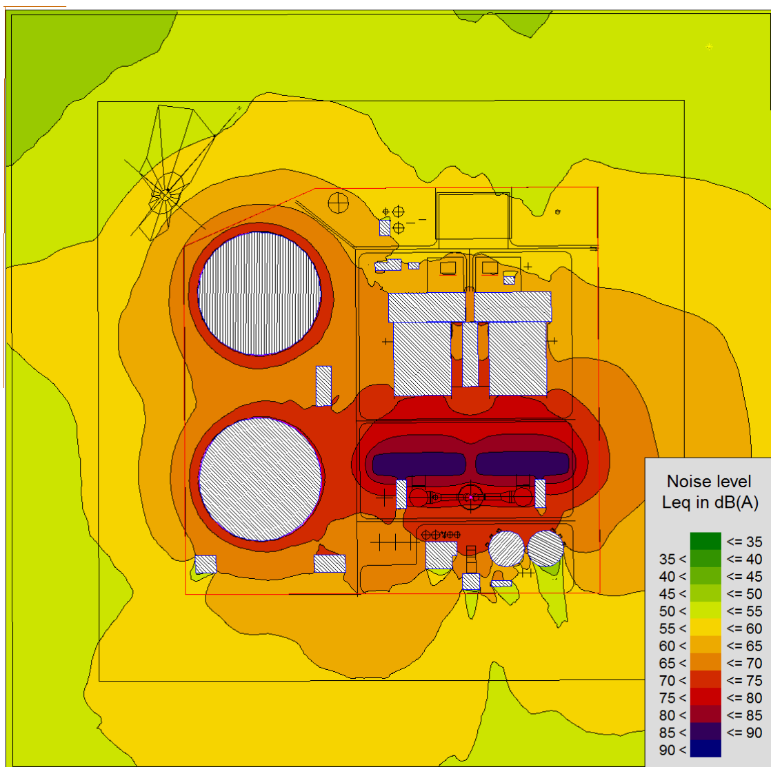
图5.4-1 在本工程现有措施正常工况下等声级线分布图
