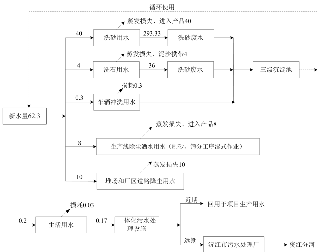
图 1-1 项目工程水平衡图 (单位: m³/d)
