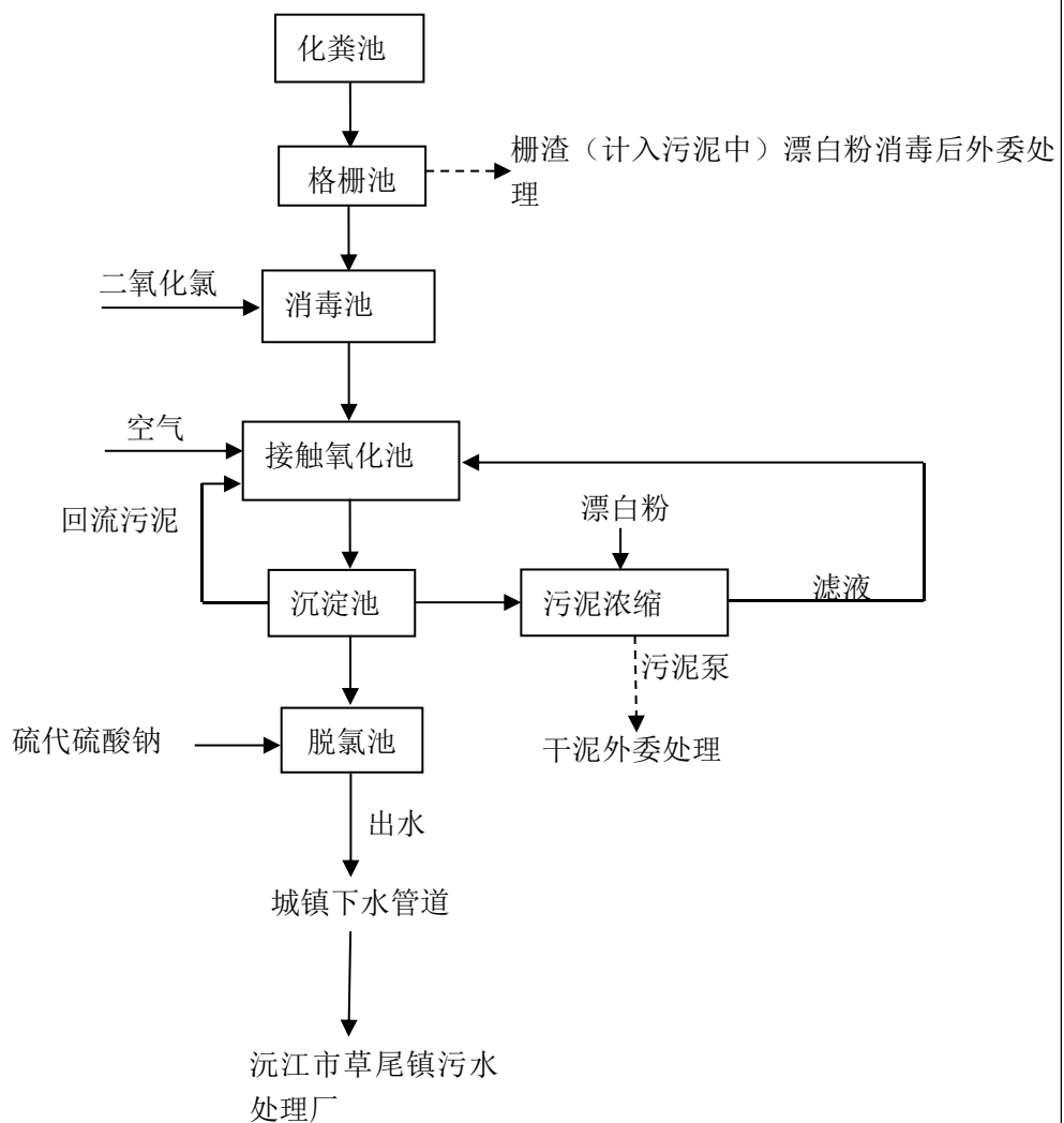
图 7-1 本项目医疗废水处理工艺流程示意图
