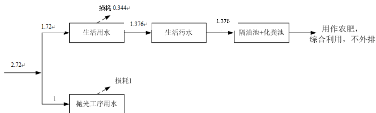
图 1-1 水平衡图（单位： \text{m}^3/\text{d} ）
