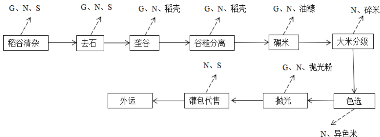
图 4-2 项目生产工艺流程及产污节点图
