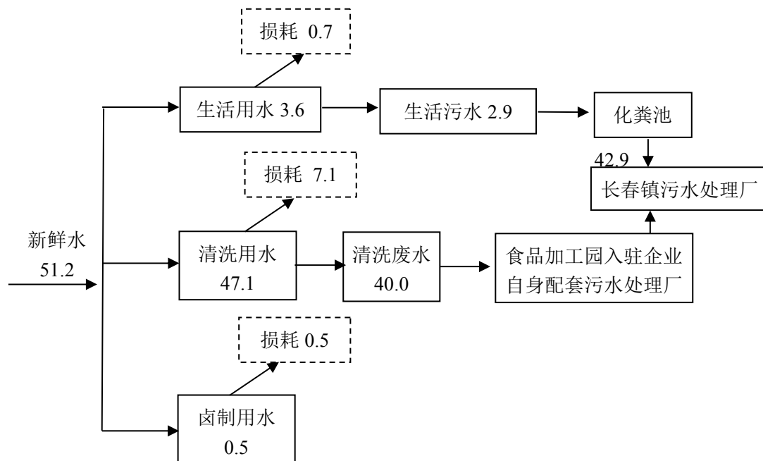
图 1-1 项目水平衡图 单位 (m³/d)
