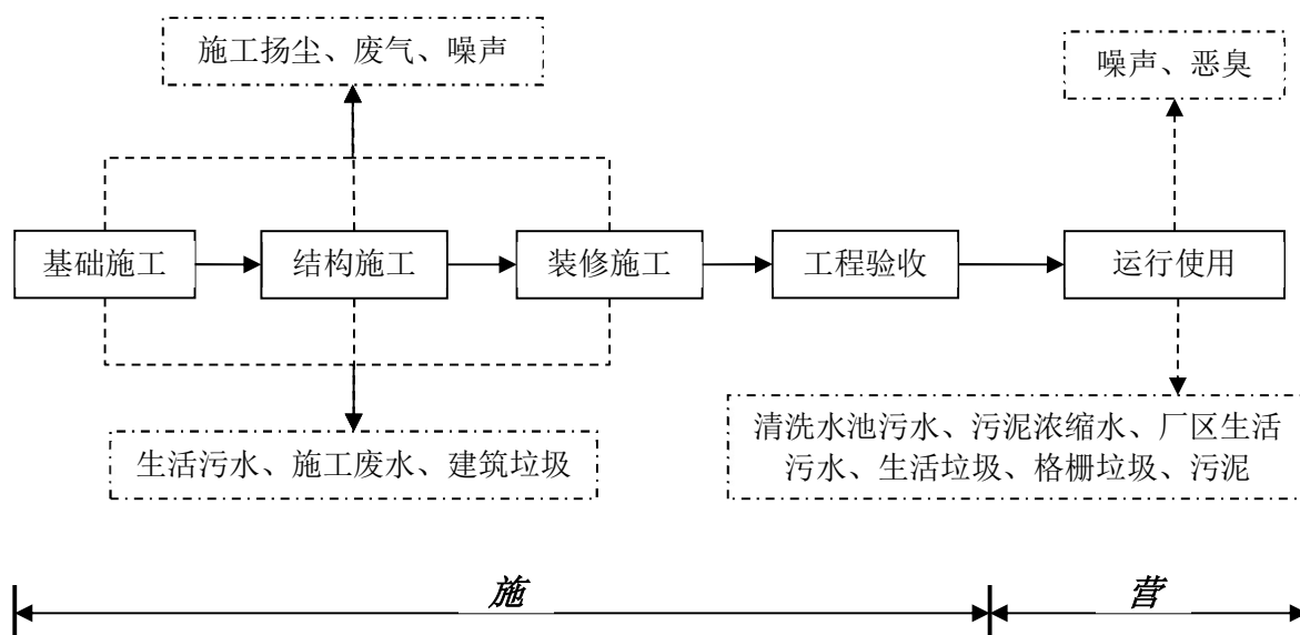
图 4-3 项目施工期、运营期流程及产物环节示意图
