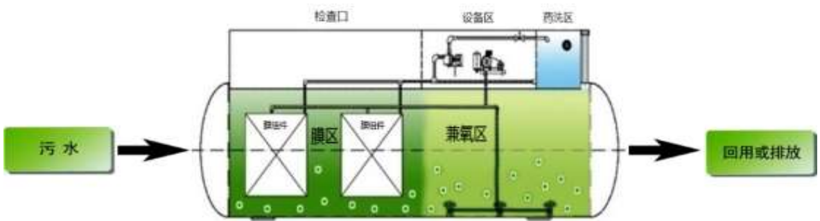
图 4-7 A 2 O+MBR 膜生物反应器内部分区图
