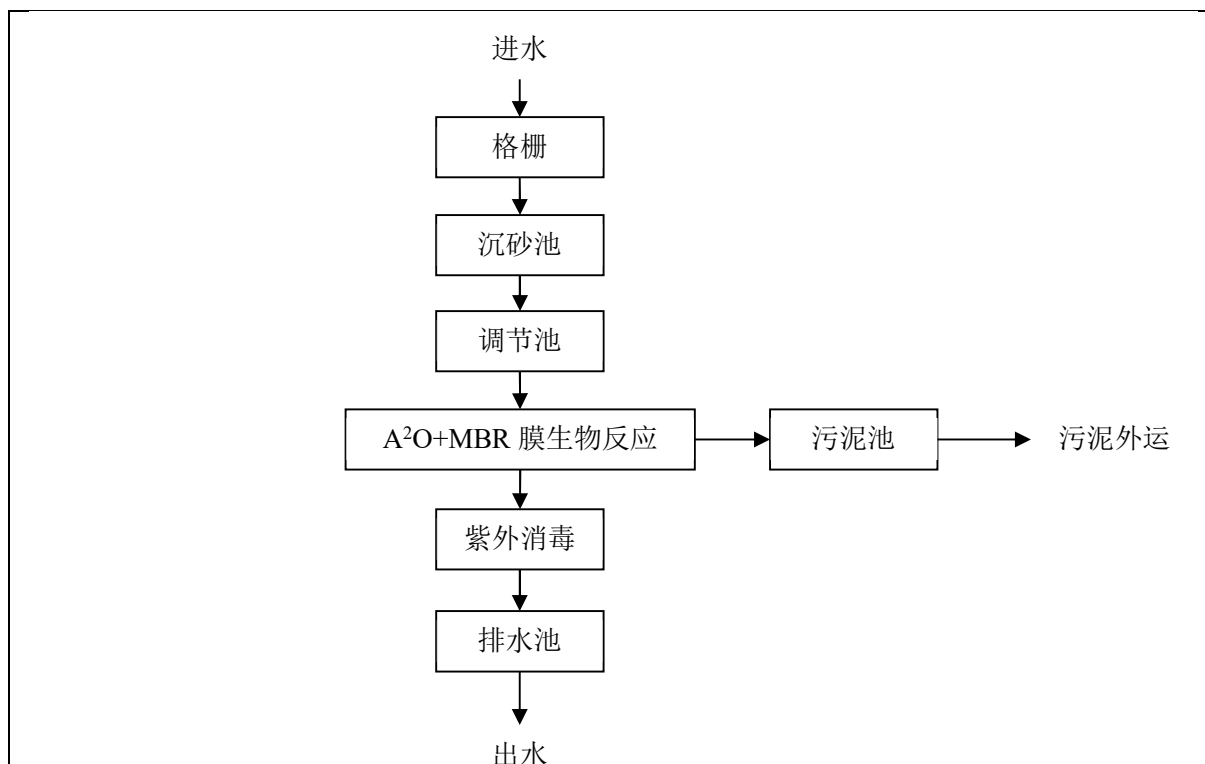
图 4-4 污水处理厂污水处理工艺流程
