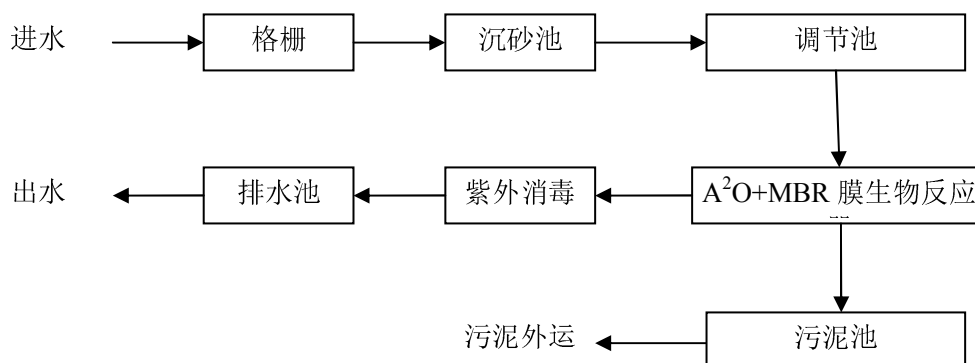
图 4-4 污水处理厂污水处理工艺流程
