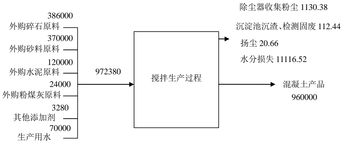
图 4-2 物料平衡图 单位 t/a
