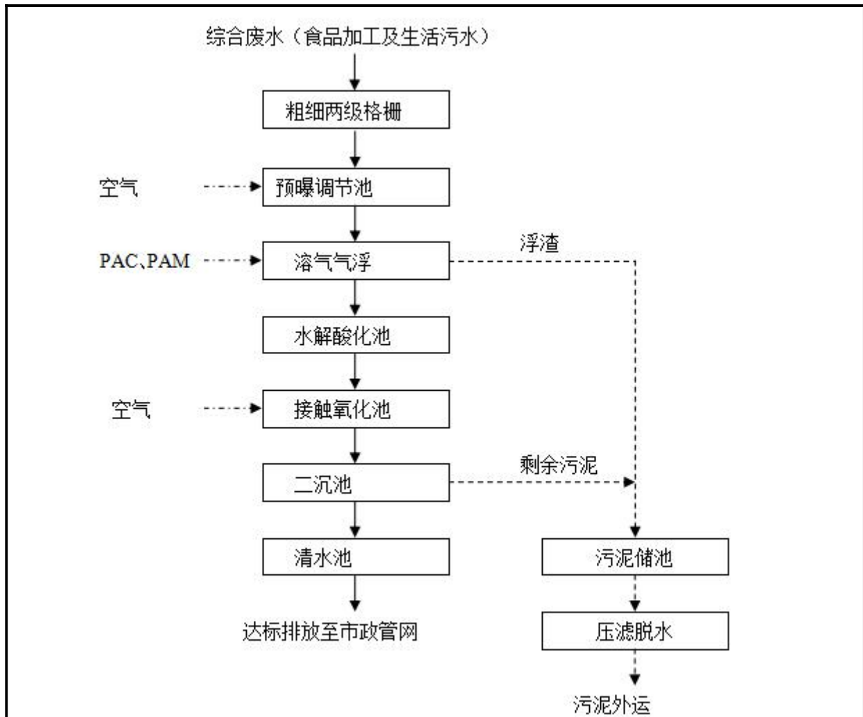
图 2-1 工艺流程及产污节点图
