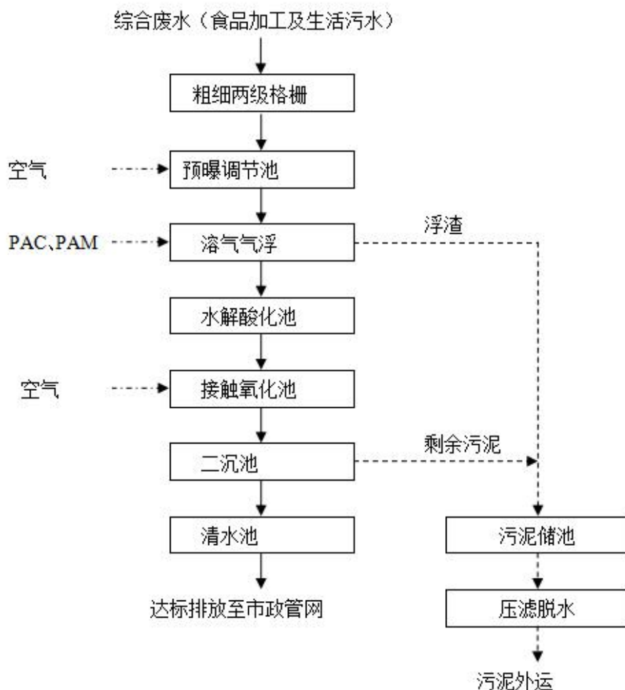
图 7-1 食品产业园污水处理站污水处理工艺流程图
