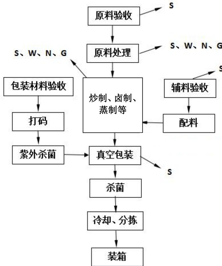
图 5-1 工艺流程图及产污节点图
