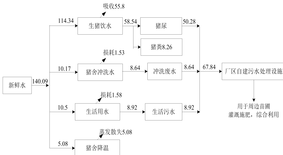
图 3.1-1 项目水平衡图 单位: \text{m}^3/\text{d}
