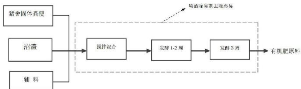
图 3.2-5 本项目堆肥工艺流程及产物节点图
