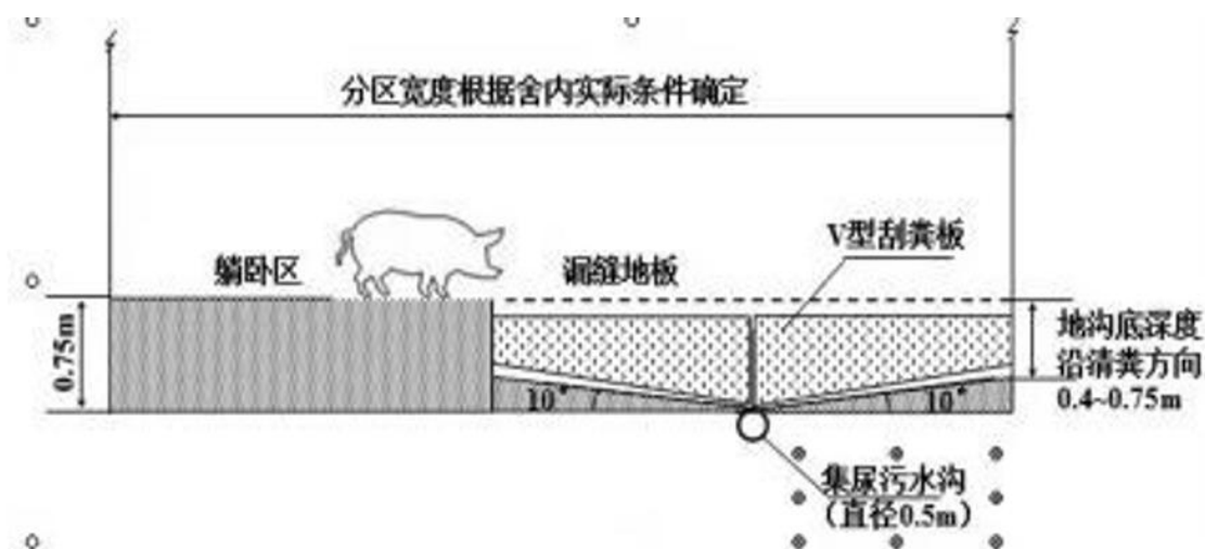
图 3.2-3 粪污处理工艺示意图
