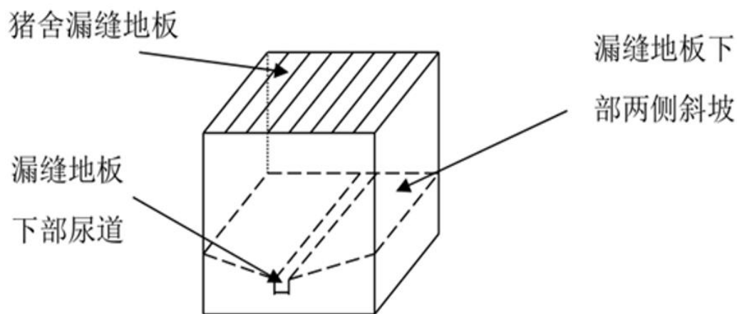
图 3.2-4 干清粪工艺猪舍下部结构视示意图
