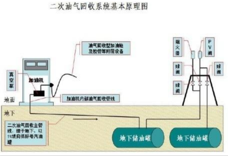
图 5-4 二次油气回收系统基本原理图
