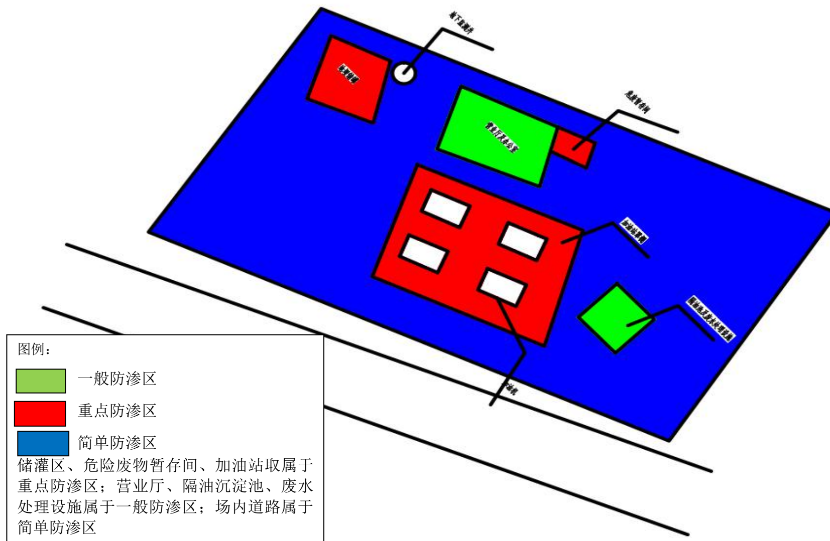
附图 2：建设项目平面布局及分区防渗图
