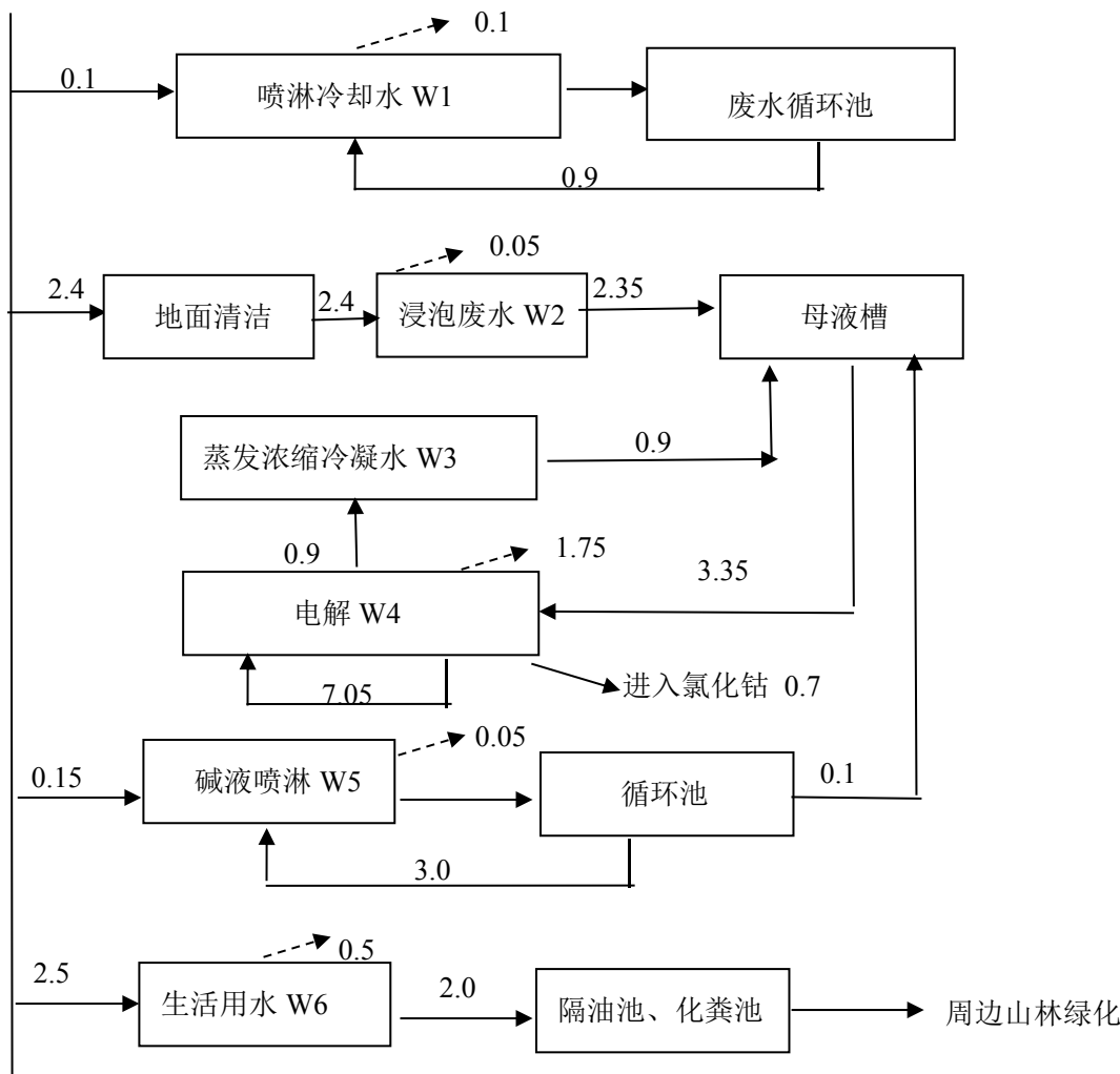
图 3.1-1 项目水平衡图 (单位: m³/d)
