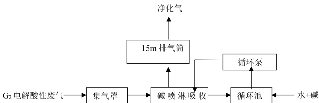
图 7.1-2 酸性废气处理工艺
