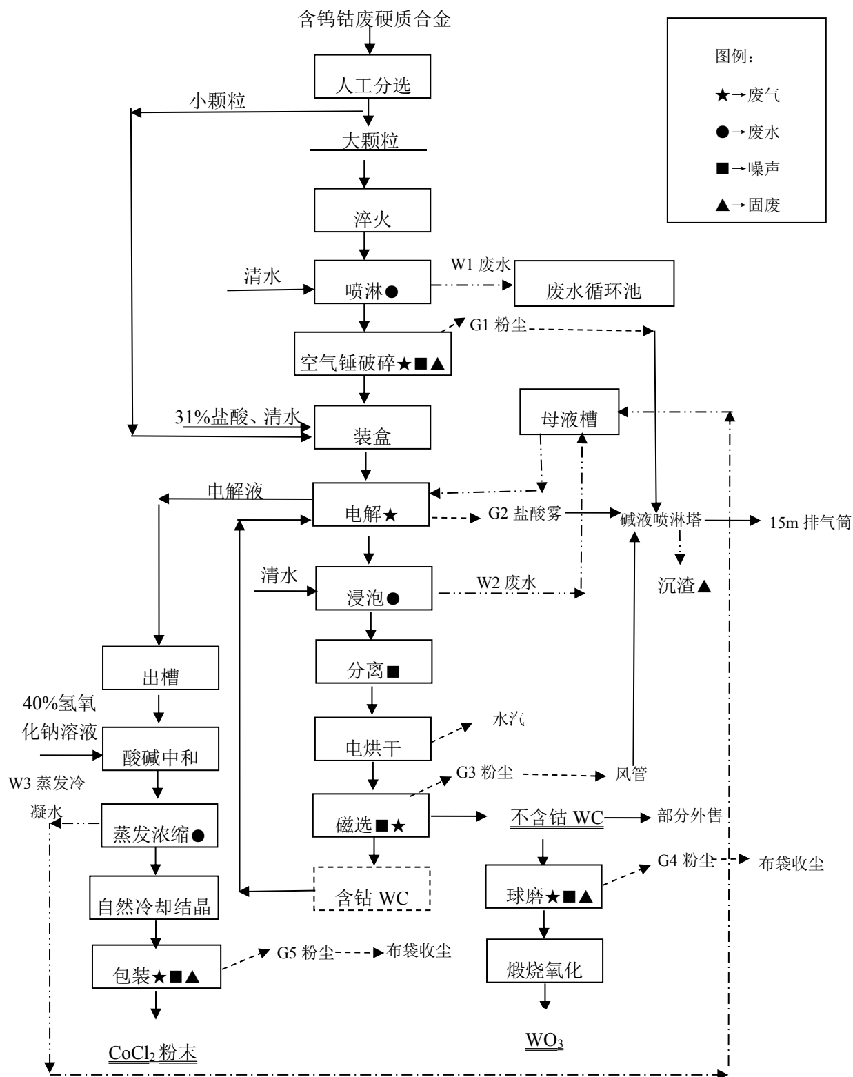
图 3.2-1 工艺流程及产污节点图
