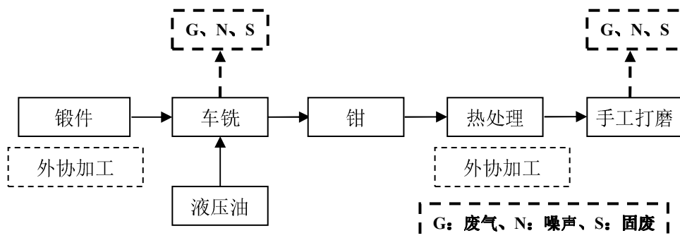
图 4-2 环类工艺流程及产污环节图
