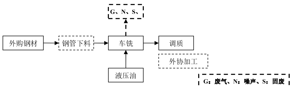
图 4-1 轴类工艺流程及产污环节图
