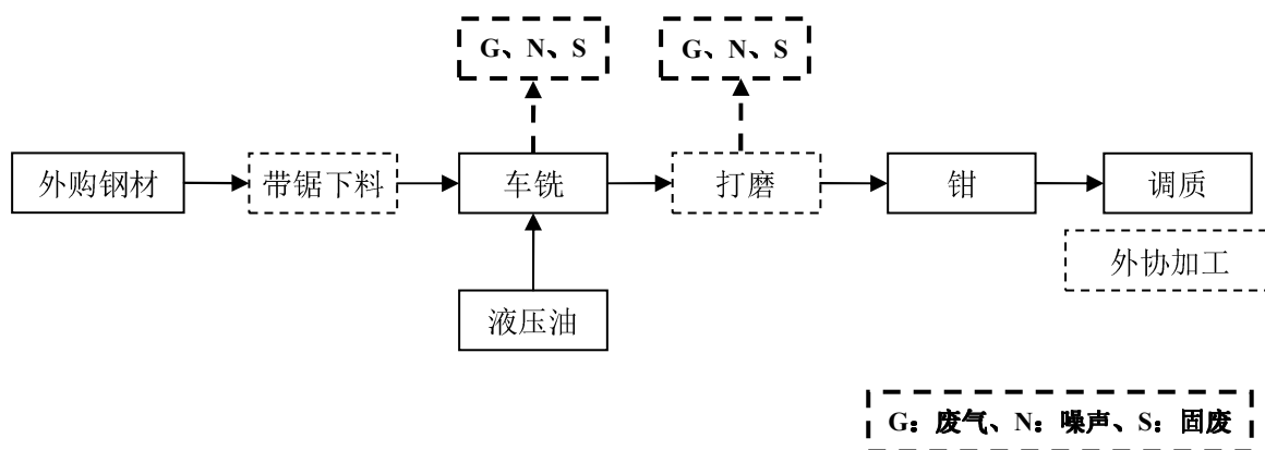
图 4-1 轴类工艺流程及产污环节图
