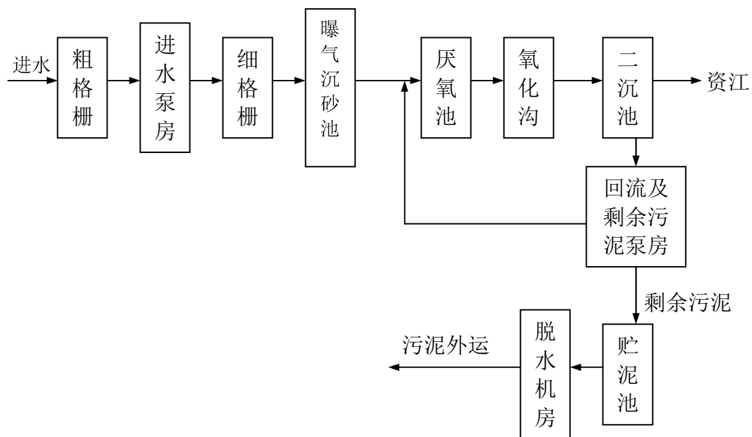
图 6-1 目前团洲污水处理厂工艺流程图
