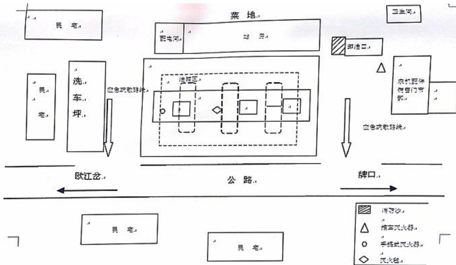
附图 2 建设项目站区平面布局图
