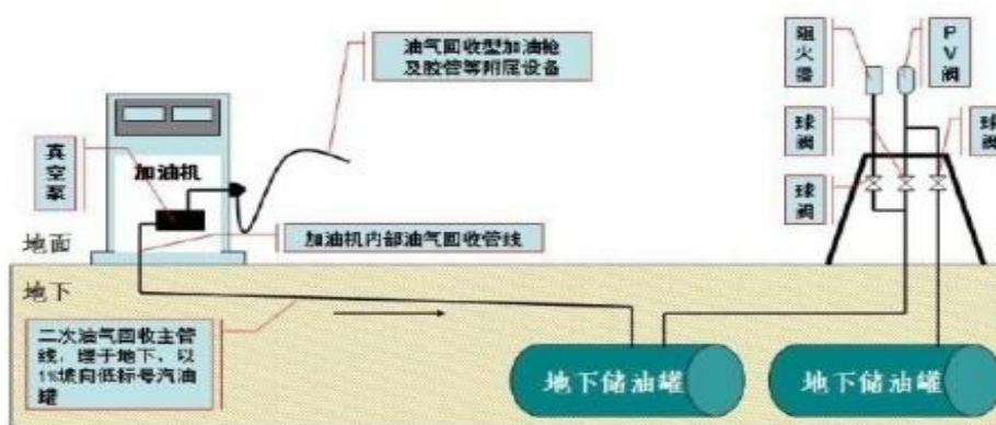
图 3.6-4 二次油气回收系统基本原理图
