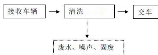
图 3.6-5 洗车工艺流程及产污节点图
