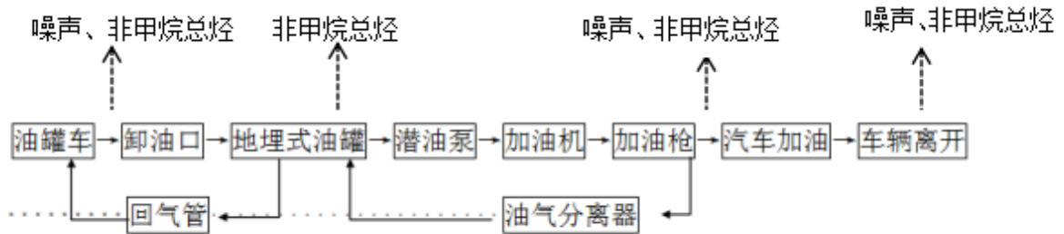
图 3-1 工艺流程及产污节点示意图
