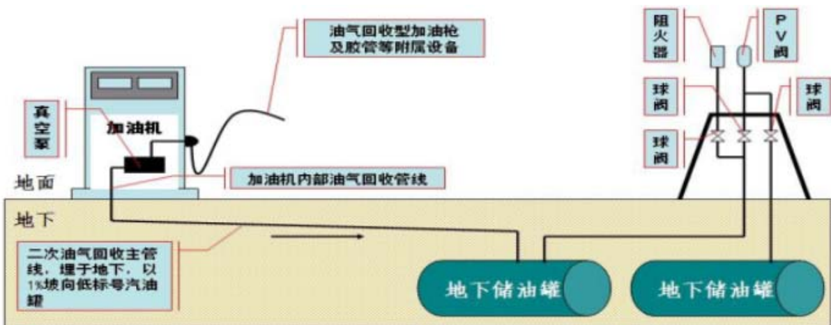
图 3-3 加油油气回收系统
