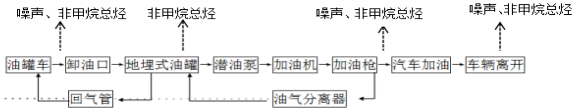
图 3-1 工艺流程及产污节点示意图
