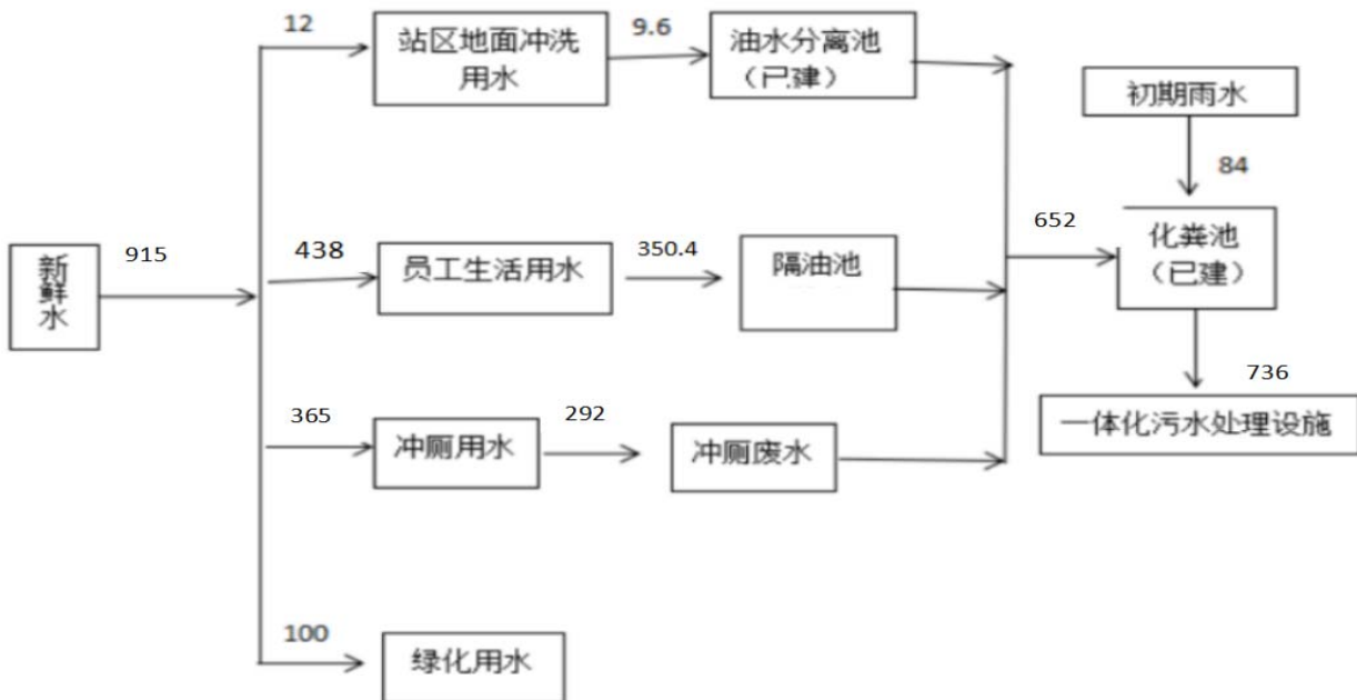
图 3-1 项目水平衡图 (t/a)
